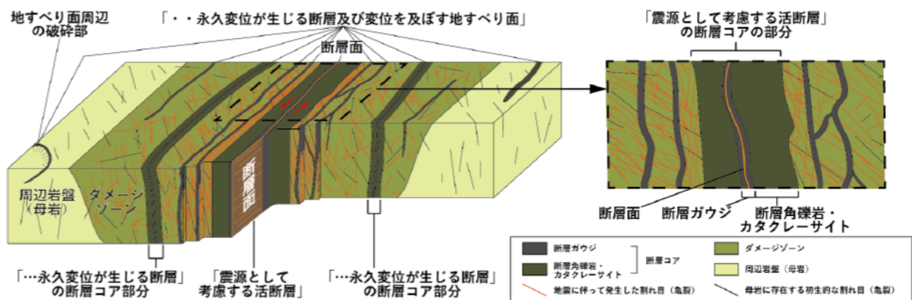
図 8 断層及びその周辺の構造の概念図 (Choi et al. 11 等を基に作成)
