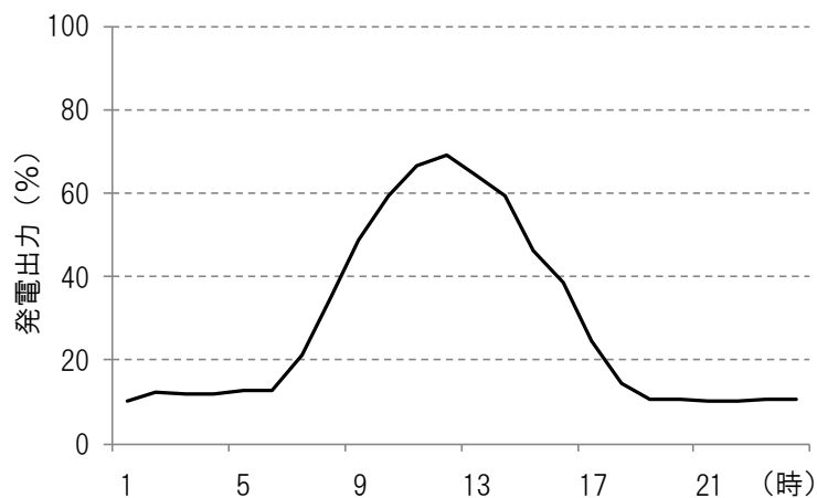
【合成出力の 2\sigma 値（晴天日）】
