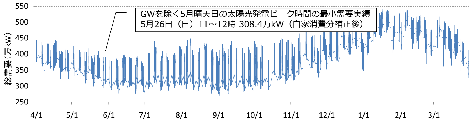
【2013年度の自社需要実績（発電受電端、離島を除く）】
