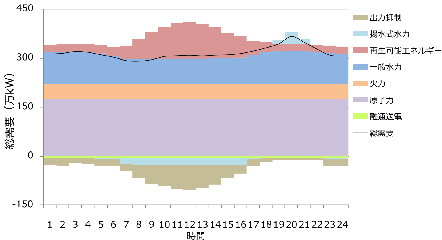
【最小需要発生日（5月26日 日曜日）のロードカーブ】
