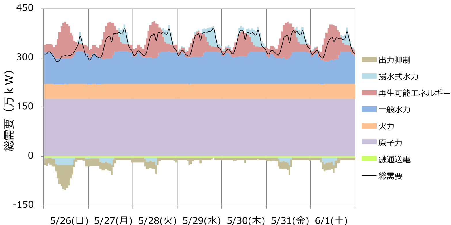
【最小需要発生日を含む1週間のロードカーブ（5月26日 日曜日～6月1日 土曜日）】
