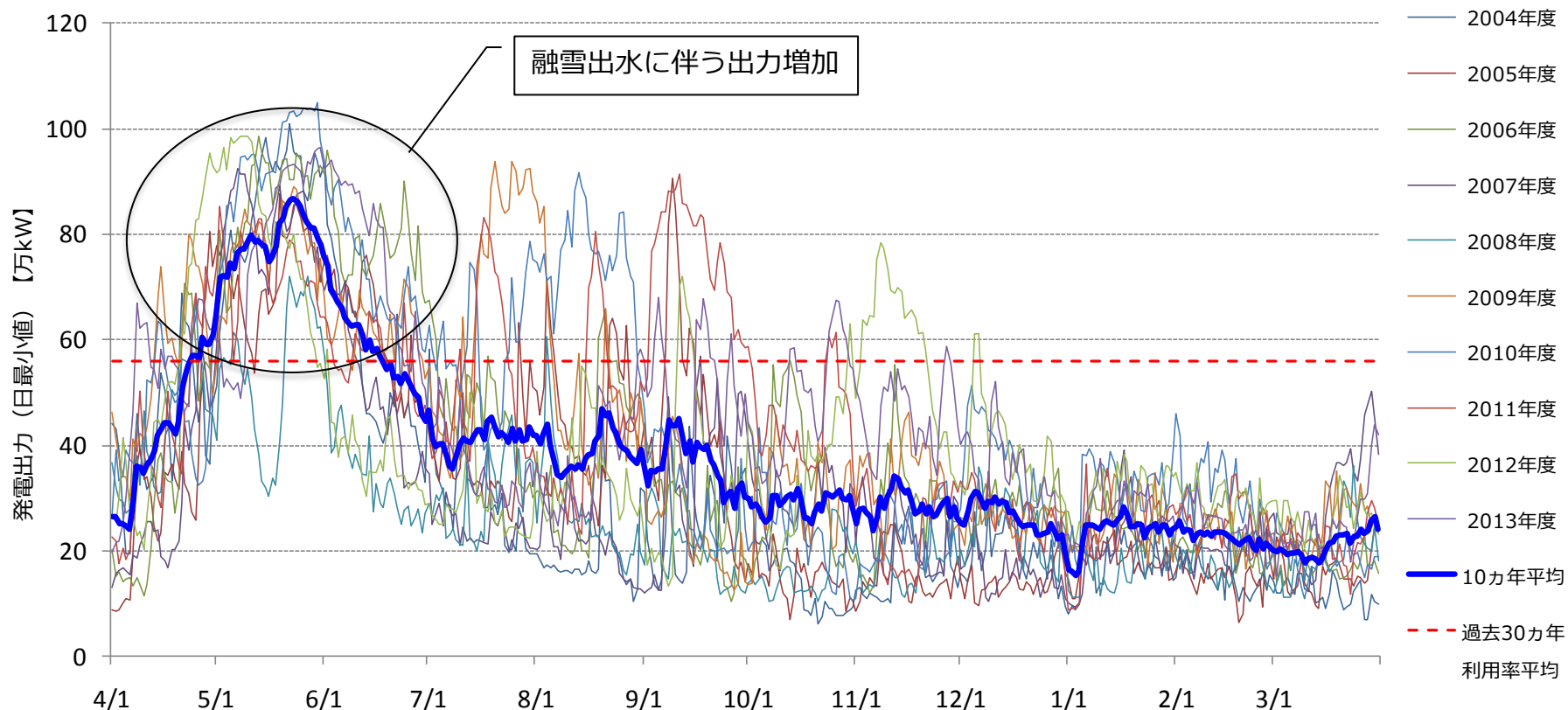
【過去10カ年の一般水力の発電実績（日最小値）】
