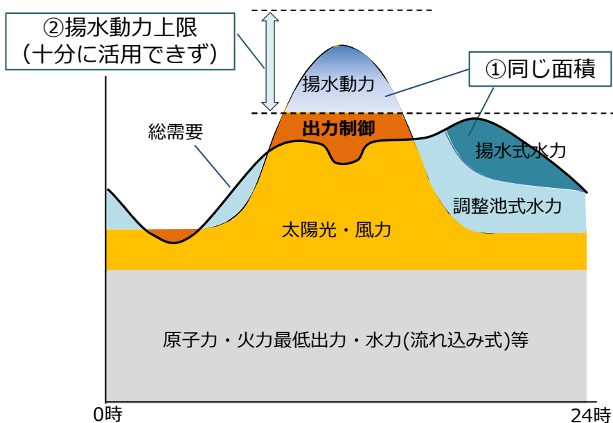
【軽負荷日のロードカーブイメージ】
