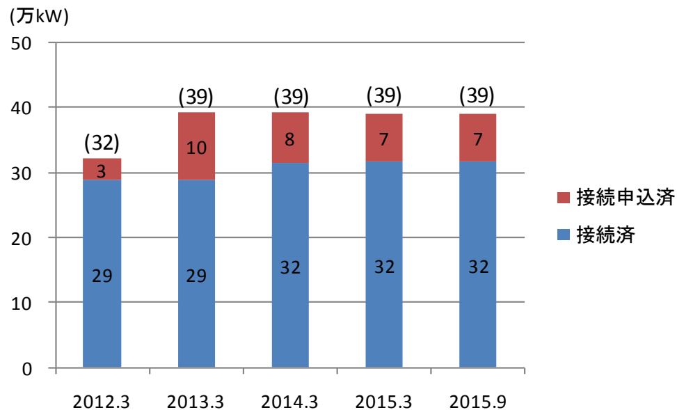
【風力発電】
