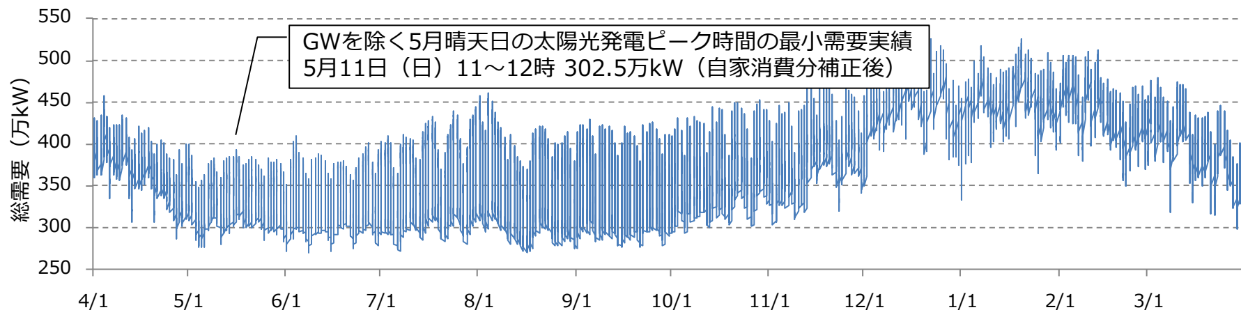
【2014年度の自社需要実績（発受電端、離島を除く）】
