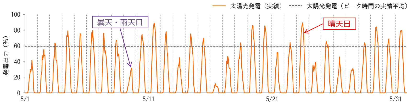
【太陽光発電の出力実績（2014年5月）】
