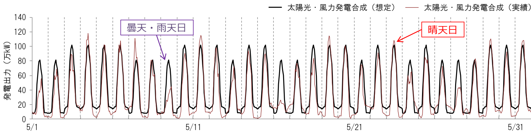
【太陽光と風力の合成出力想定】
