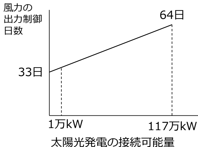
【風力の出力制御日数】 (風力発電36万kWを前提)
