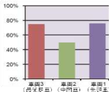
空気抵抗低減値(車間距離4m時)
