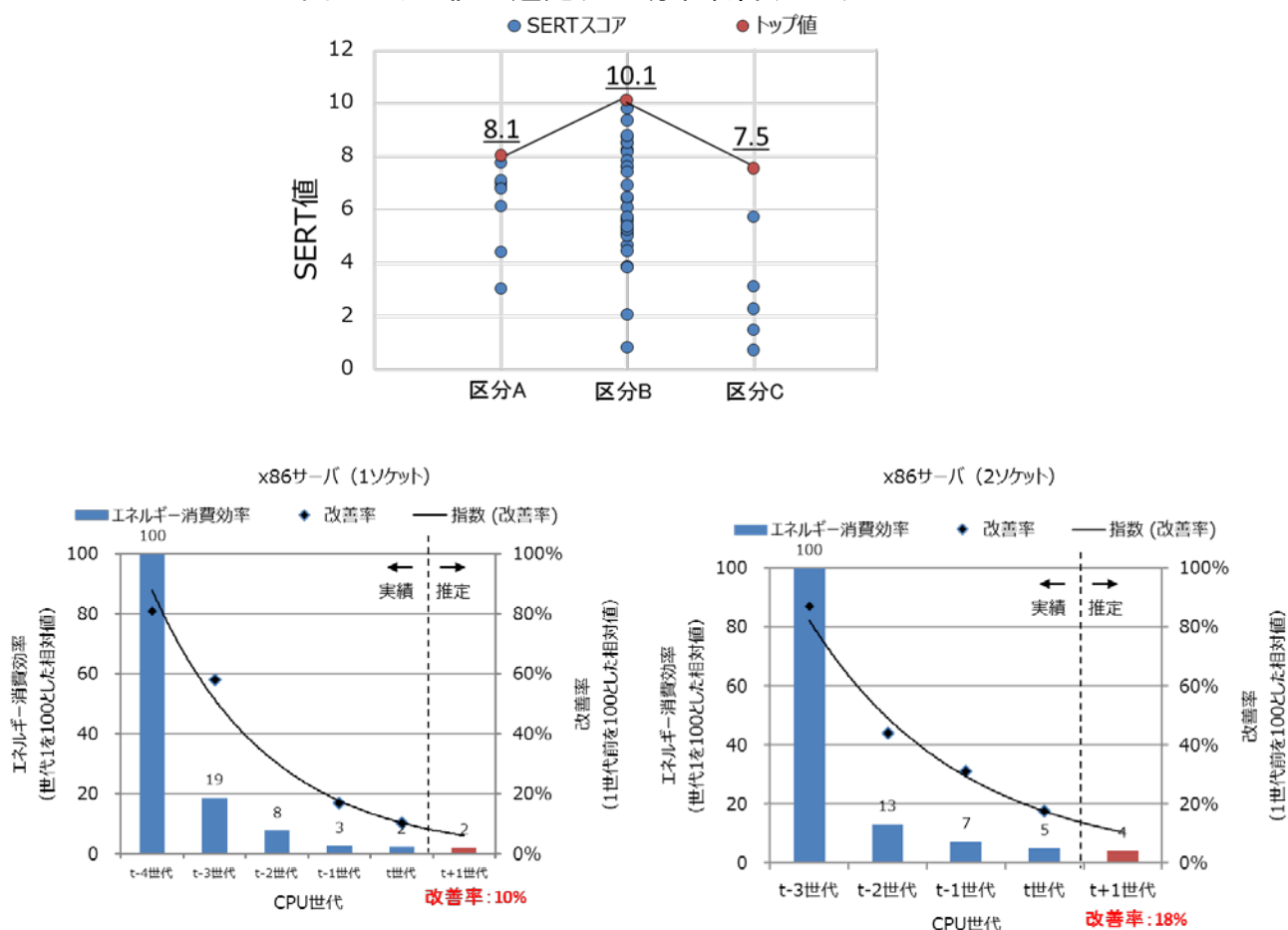
図1. トップ値の選定及び効率改善 (x86)
