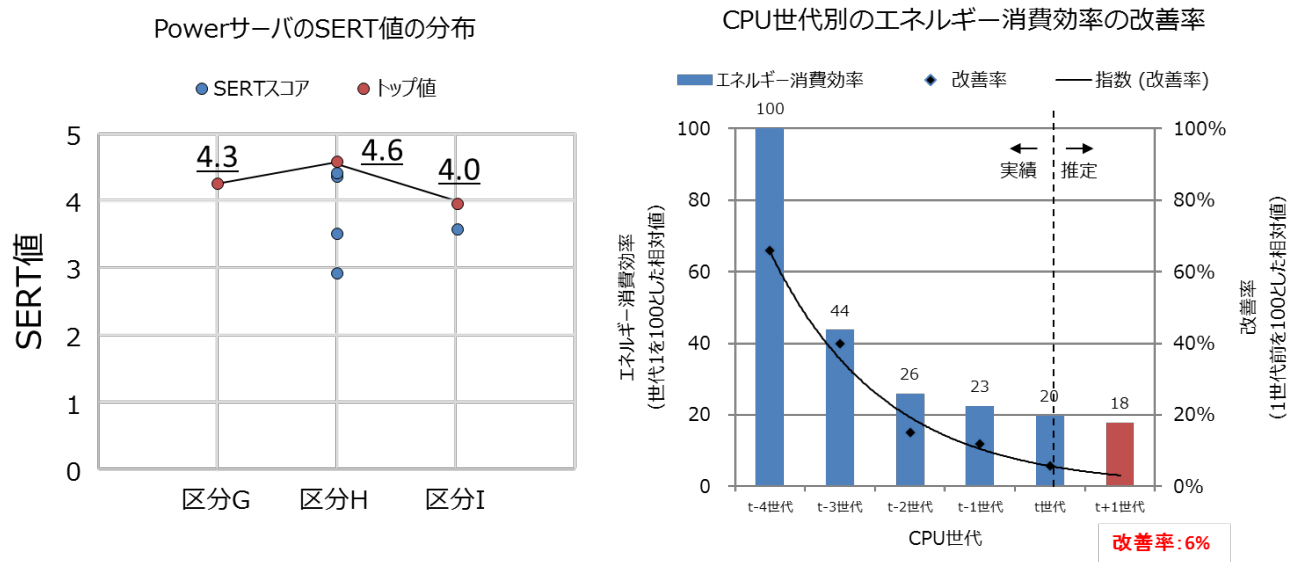
図3. トップ値の選定及び効率改善 (Power)
