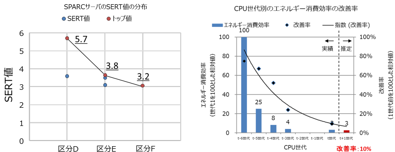
図2. トップ値の選定及び効率改善 (SPARC)
