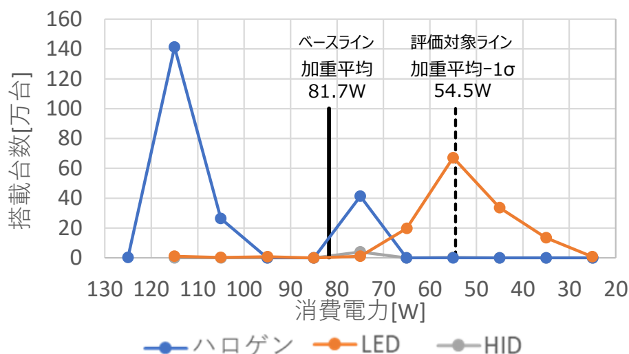
図2 評価対象ラインとベースラインのイメージ (2016年度におけるライト（ロービーム）の例) (提供) 一般社団法人日本自動車工業会
