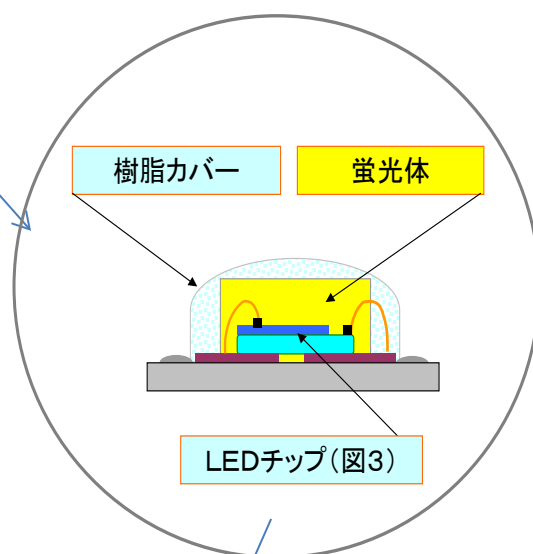
図 2. LEDパッケージ
