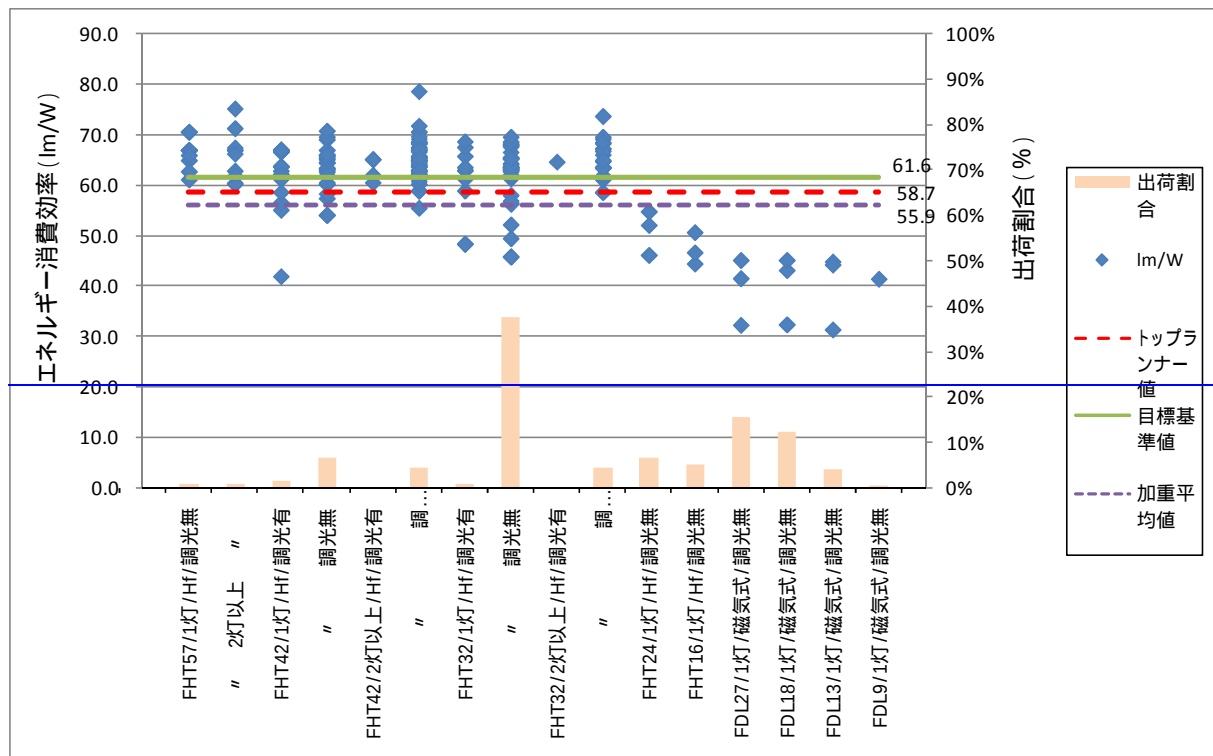
図3．区分（施設用であって、2本管形以外のコンパクト形蛍光灯を使用するもの）の目標基準値
