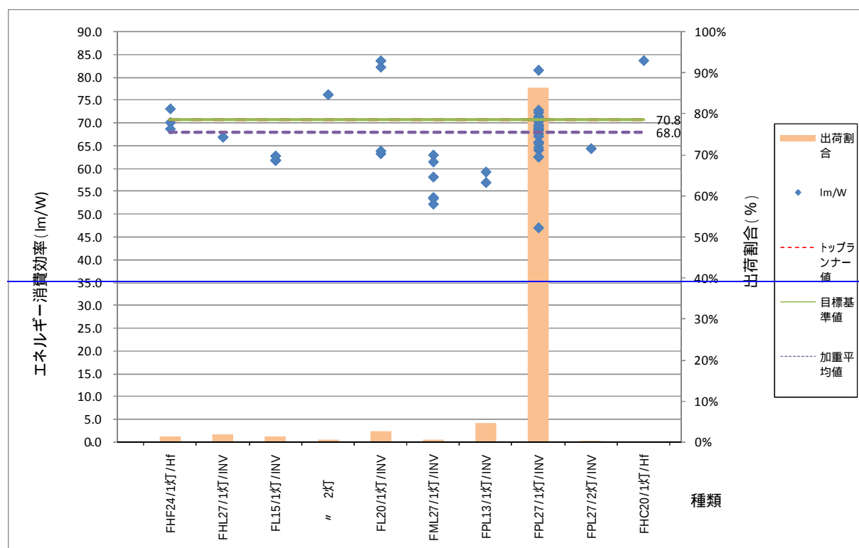
図6. 区分 (卓上スタンドであって、直管形またはコンパクト形蛍光ランプを使用するもの) の目標基準値
