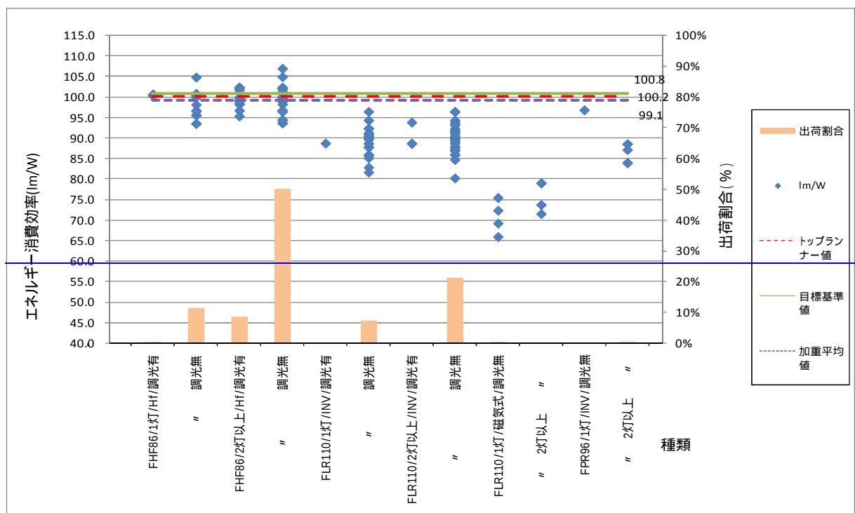
図1．区分（施設用であって、ランプの大きさが86以上の直管形蛍光ランプまたは2本管形のコンパクト形蛍光ランプを使用するもの）の目標基準値
