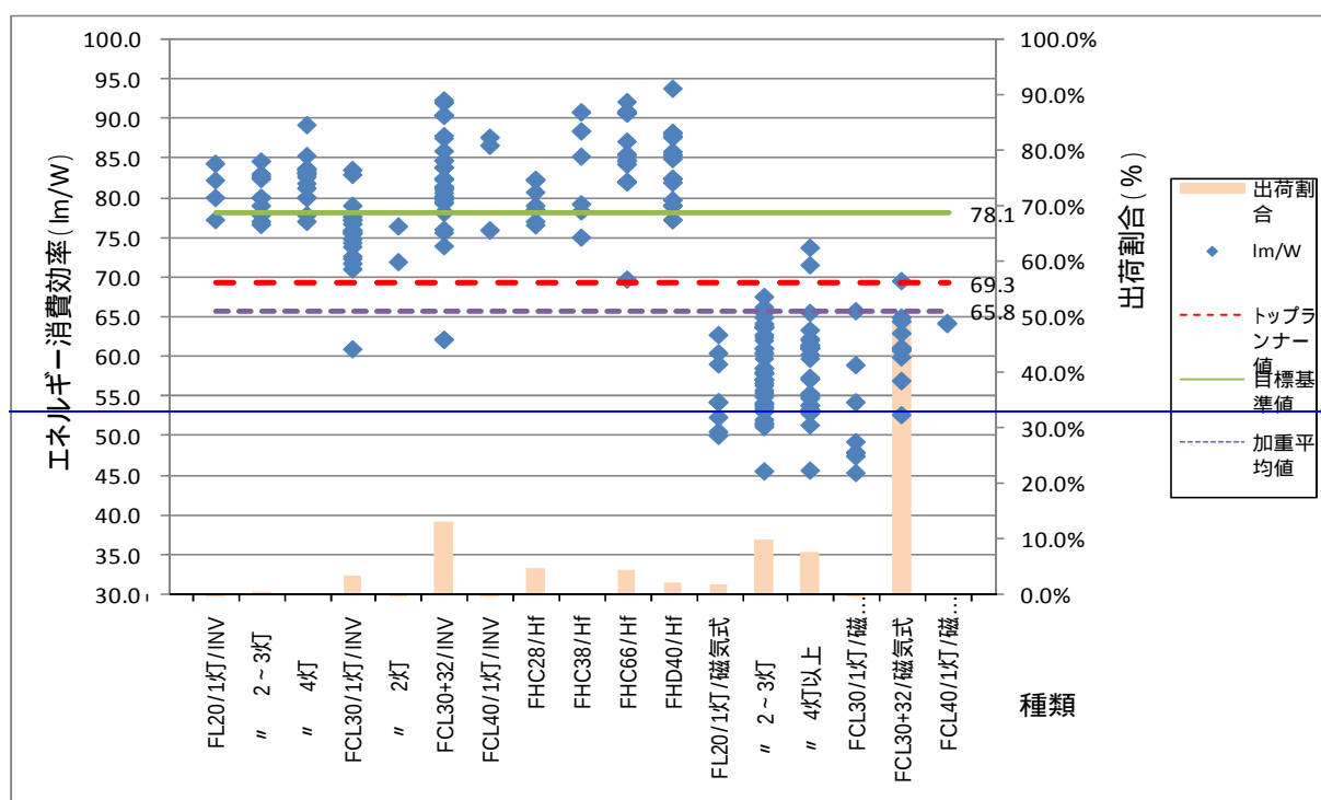
図5. 区分 (家庭用であって、ランプの大きさの総和が70未満の環形または直管形蛍光ランプを使用するもの及びランプの大きさの総和が70以上であって、ランプの大きさが20の直管形蛍光ランプを使用するもの)の目標基準値
