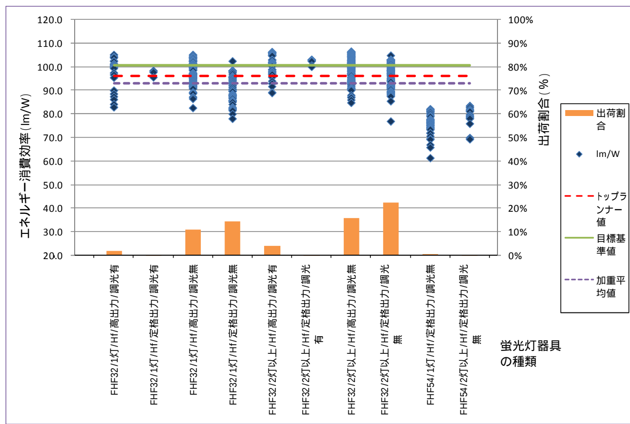
図2 区分 のF H Fランプを使用する蛍光灯器具のエネルギー消費効率
