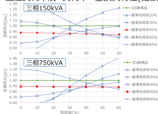
最適負荷率別 負荷率－全損失特性(指数)
