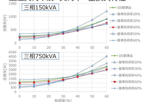
最適負荷率別 負荷率－全損失特性
