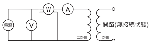
図1 単相変圧器の無負荷損試験回路
