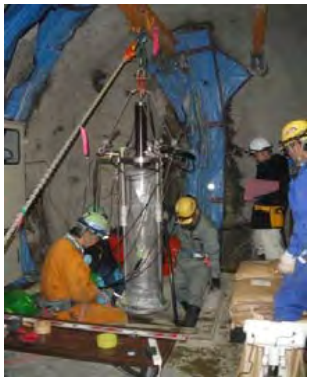
溶接部腐食試験装置の設置作業
