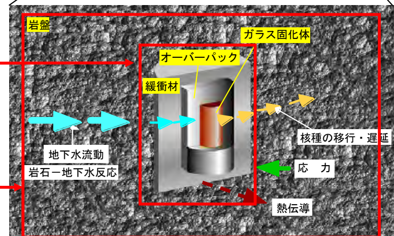
人工バリア周辺で生じる複合現象
