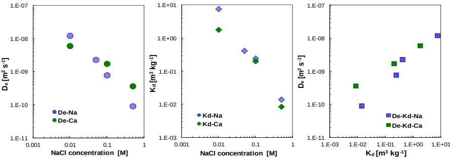
図2 圧縮モンモリロナイト中のSrの核種移行データ（収着分配係数Kd,実効拡散係数De）の塩濃度依存性
