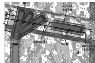
廃棄体（使用済燃料）の定置方法を 考慮した処分坑の検討
