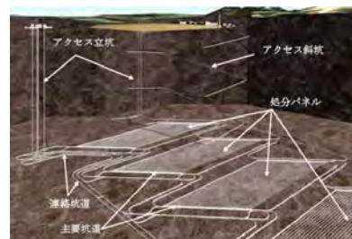
地層処分施設の設計概念 (ガラス固化体の場合)
