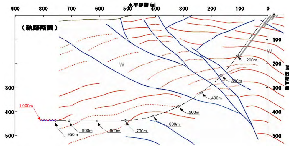
コントロール掘削実績(HCD-3孔井：上幌延サイト)
