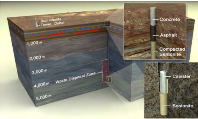
図2 超深孔処分の検討例（米国）
