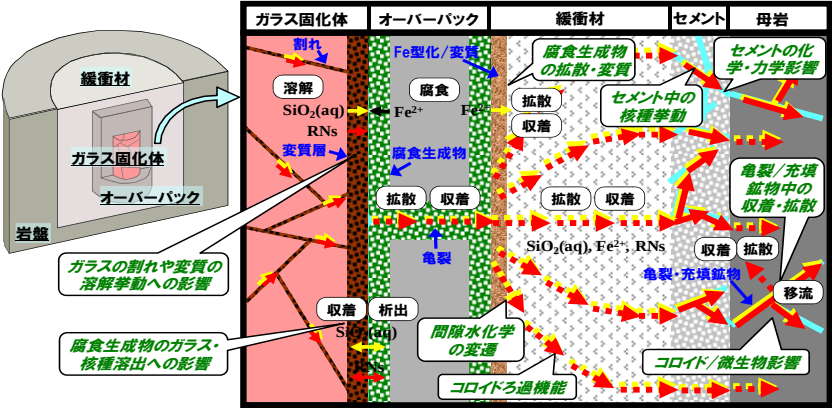
図1 ニアフィールドにおいて時間的変遷に伴い発生する現象（図中吹き出し）と核種の移行経路（図中矢印）の概念図
