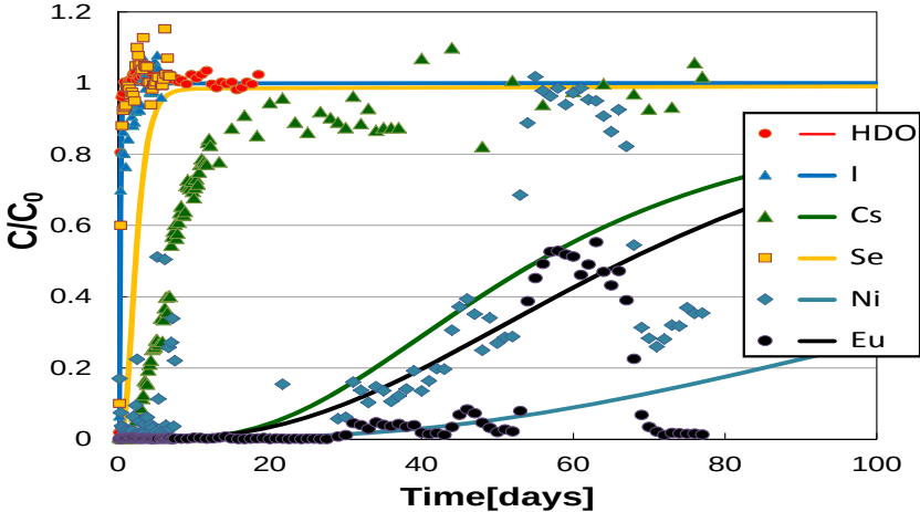
図3 花崗岩割れ目中の通液試験の結果（図中プロット）と解析結果（図中実線）の比較
