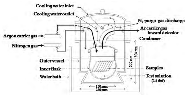
水素測定法によるハル・エンドピースの長期腐食試験
