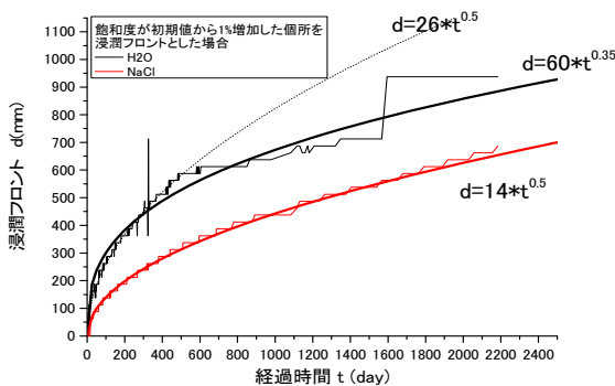
緩衝材中の浸潤フロントの進展
