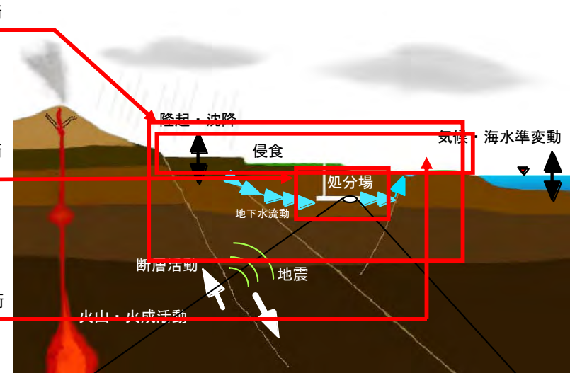
地層処分の概念と想定される天然現象
