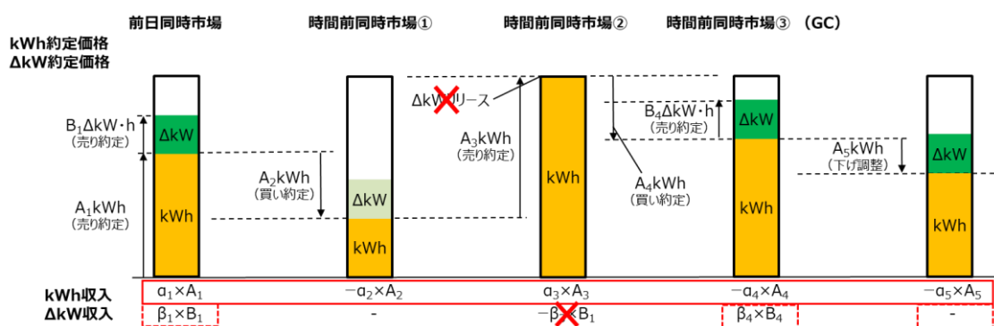
図 26 約定点近辺にある電源の約定推移と収入（例 2）
