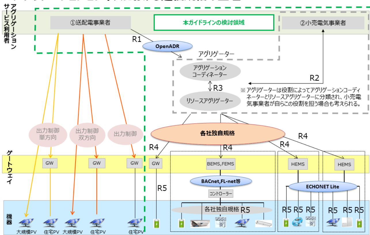
図1 ERABシステムにおけるインターフェース
