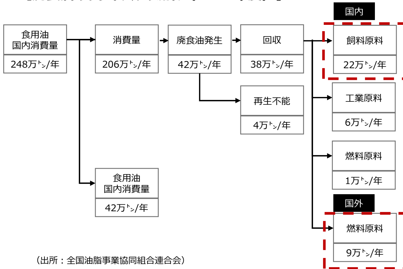
【廃食油のリサイクルの流れ（2020年度）】
