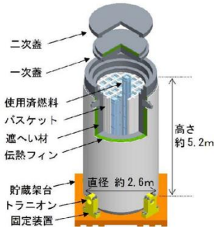
【乾式貯蔵容器】
