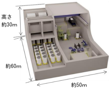
【乾式貯蔵建屋】
