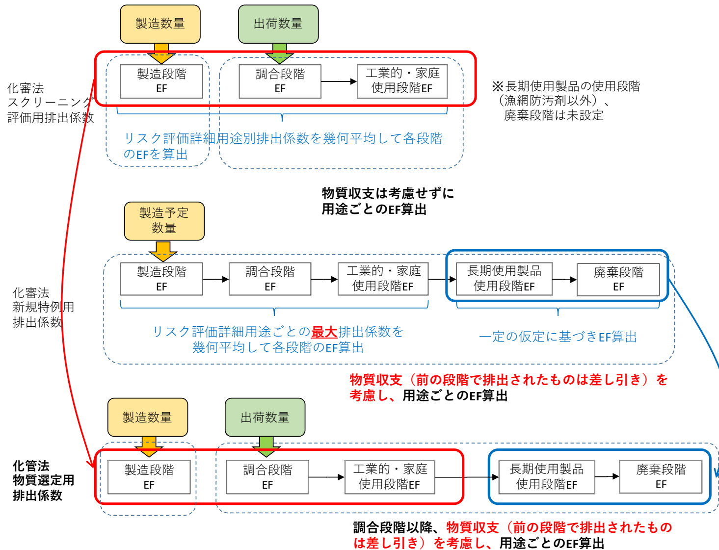
図 3 取りまとめにおける化管法物質選定用排出係数設定方針
