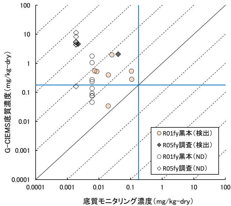
図 3 G-CIEMS 推計底質濃度（令和 2 年度実績）と、底質モニタリング濃度（黒本調査（令和元年度）、令和 5 年度優先評価化学物質の環境残留状況把握調査）との比較
