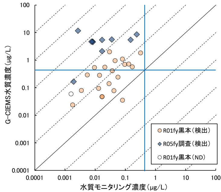
図 2 G-CIEMS 推計水質濃度（令和 2 年度実績）と、水質モニタリング濃度（黒本調査（令和元年度）、令和 5 年度優先評価化学物質の環境残留状況把握調査）との比較
