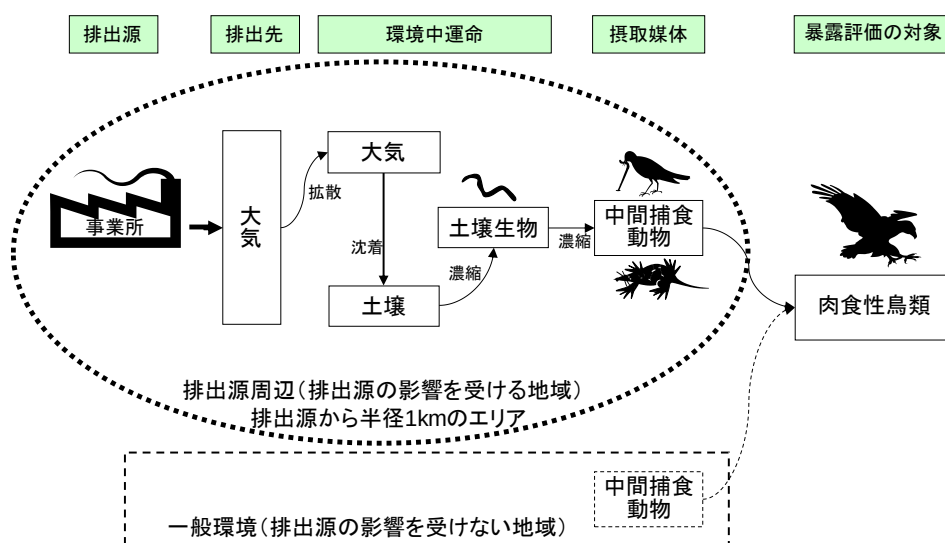
図 6-1 肉食性鳥類の暴露シナリオ
