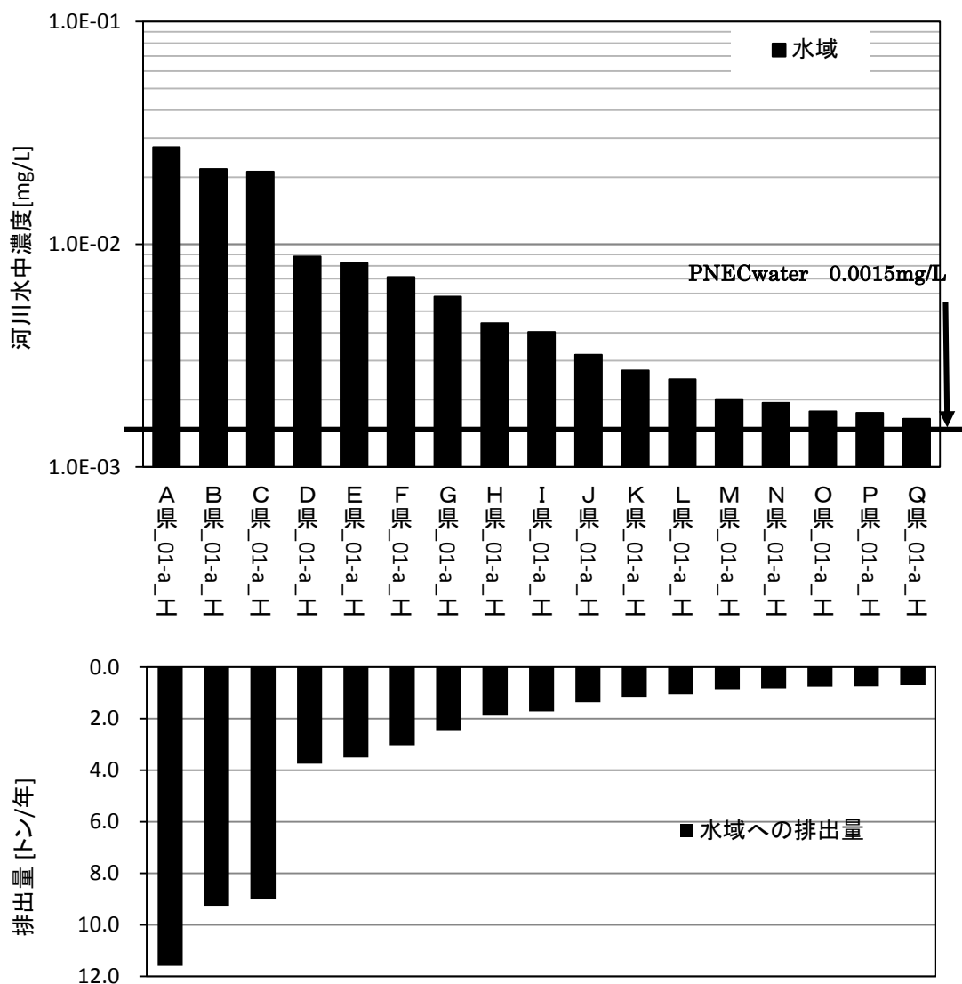
1 2 3 図 5-3 化審法届出情報に基づく仮想的な排出源(水域)の推計排出量に対する河川水中濃度 4 5
