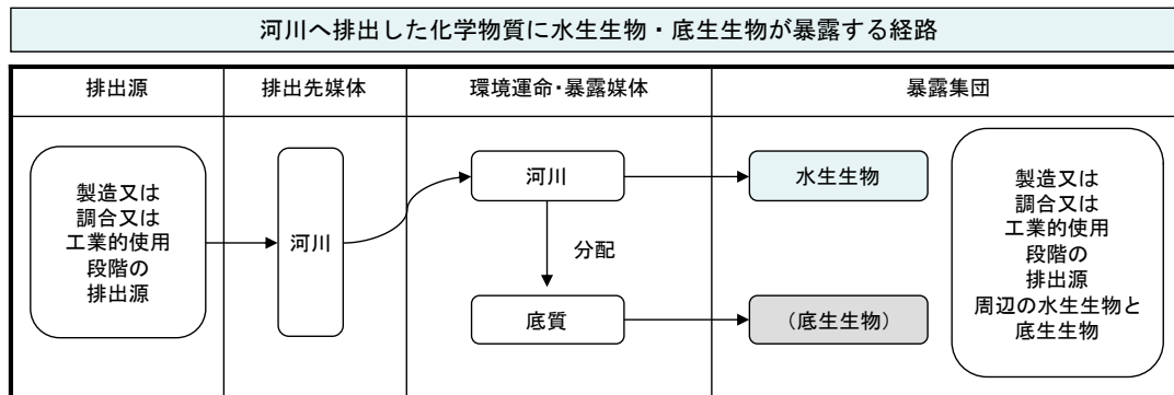
9 10 図 5-2 排出源ごとの暴露シナリオ(logPow が 3 以上の物質の場合は底生生物も対象)
