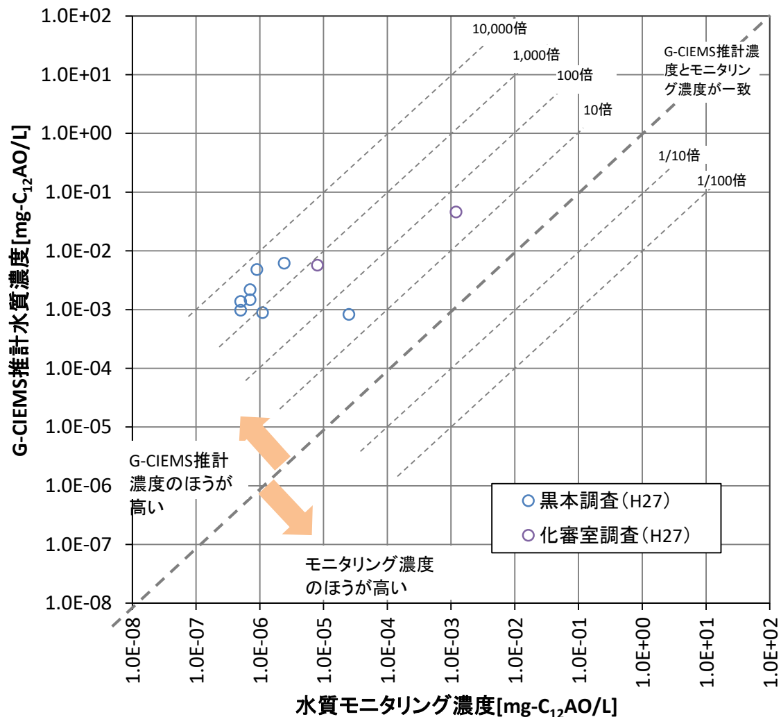
6 図 3 G-CIEMS 推計水質濃度 (PRTR、平成 26 年度) と
