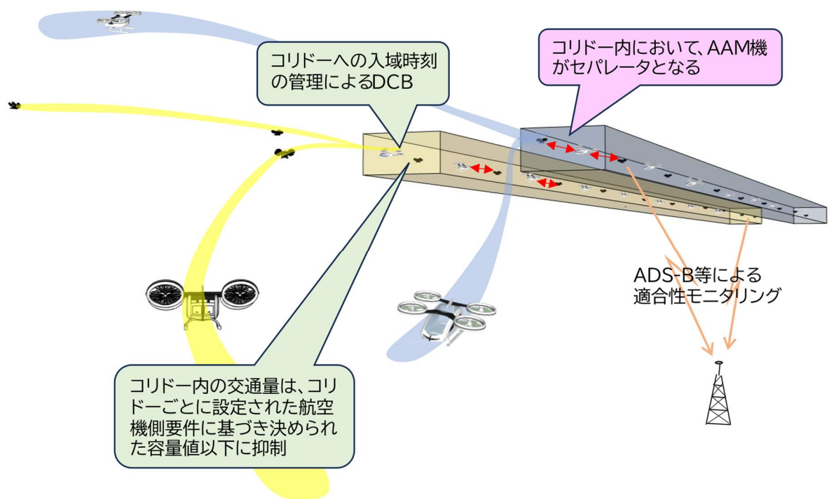
図 4-4 フェーズ 2 の後半の自動化・自律化した AAM 機の AAM コリドールの概念図
