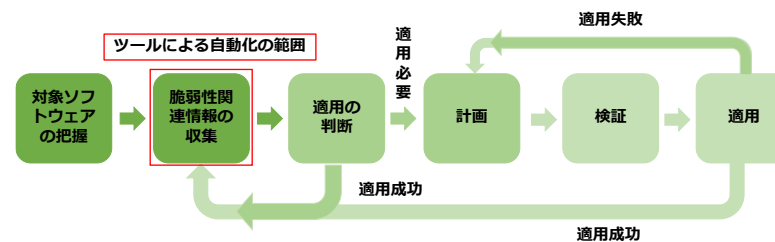
図 3-8 脆弱性対策のフロー（例） 39
