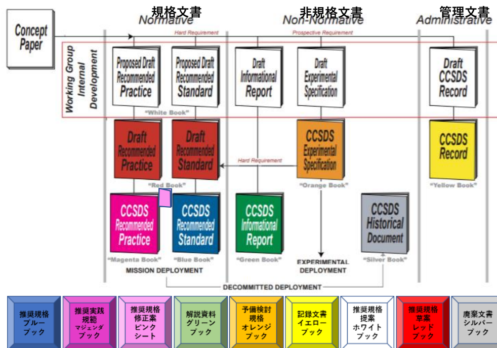
図 3-7 CCSDS の文書の分類 26, 27
