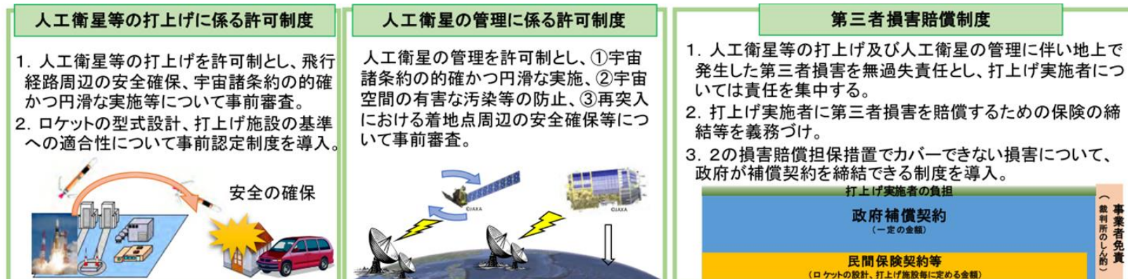
図 3-4 人工衛星等の打上げ及び人工衛星の管理に関する法律の主な内容 19
