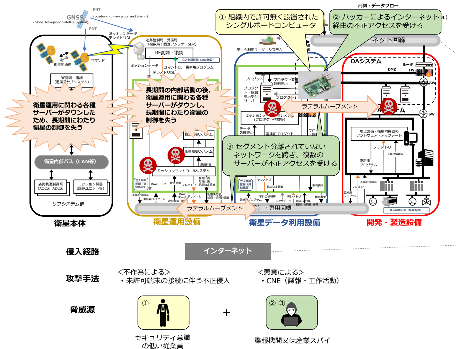
図 2-8 リスクシナリオ例3：衛星データ利用設備へのサイバー攻撃による衛星制御の喪失
