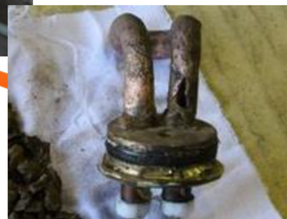
制御装置端子部の腐食
