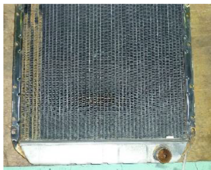
ラジエータ フィンの劣化
