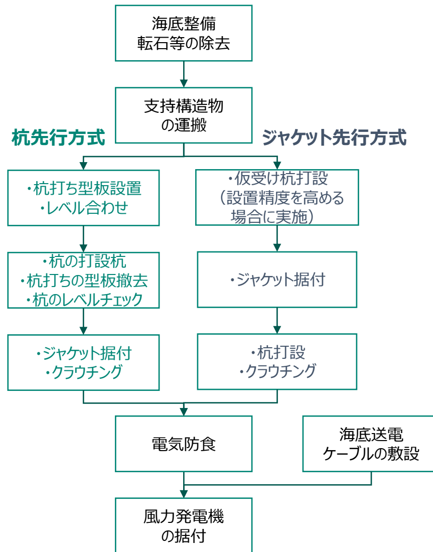
図 ジャケット式の施工の流れ
