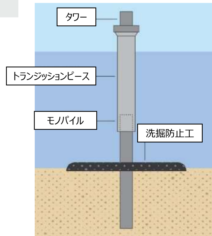
図 モノパイル式のイメージ図
