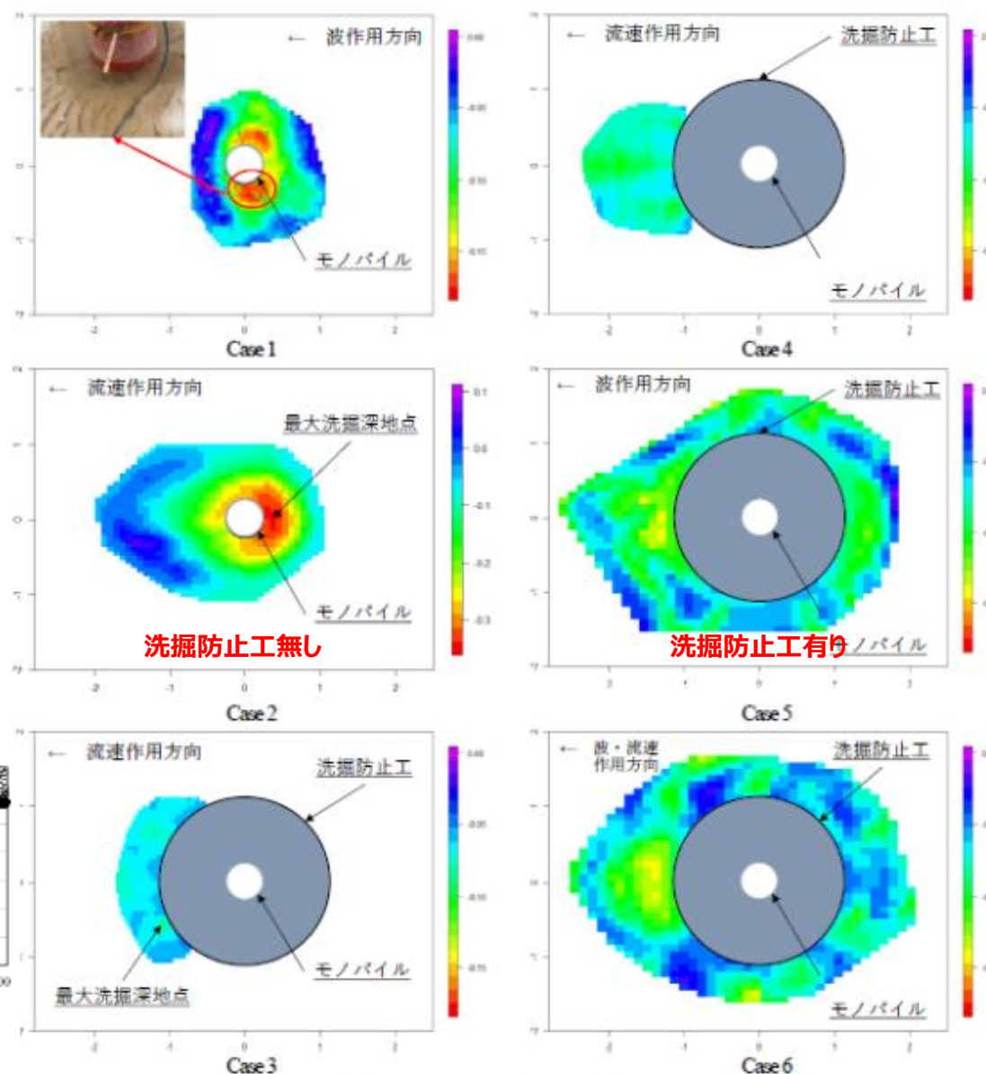
図5 各ケースの最終洗掘深 (単位: m)
