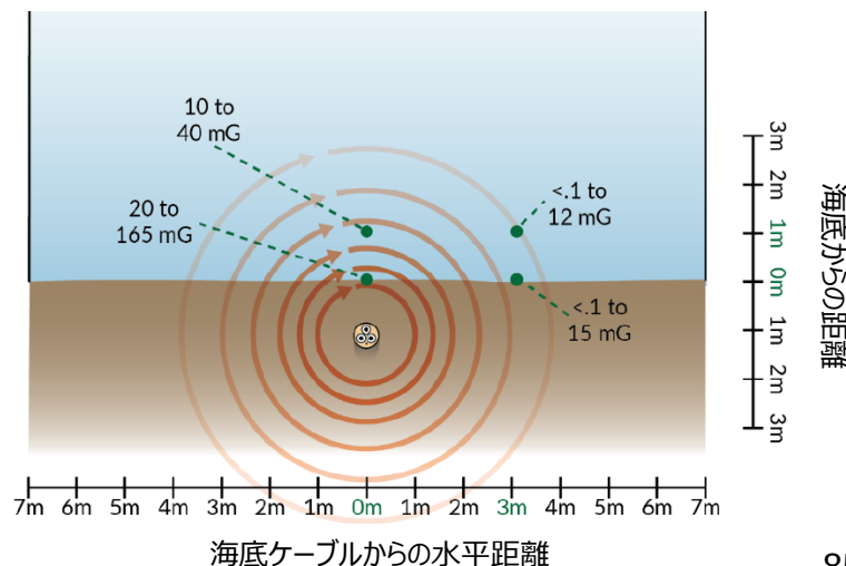
エクスポートケーブルの磁界レベル（1m埋設した場合）
