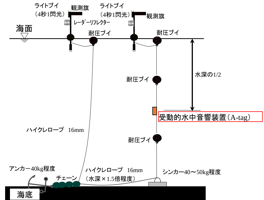
受動的水中音響装置の設置イメージ
