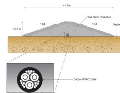
ケーブルを被覆した場合の断面
