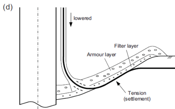
(d) 海底ケーブル海底送電線及び通信ケーブル 敷設後に洗掘防止工を施す場合
