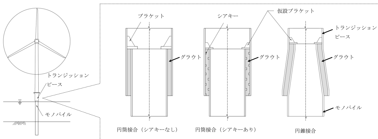
図-解 4.9.1 モノパイル構造におけるグラウト接合部の例 1)
