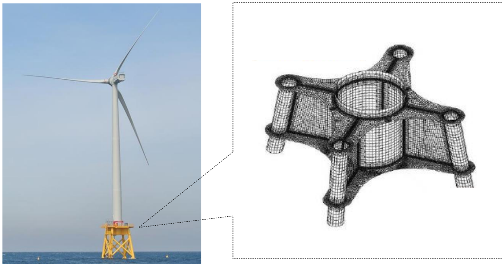
図-解 4.9.2 ジャケット構造における鋼構造接合部の例 2)、3)
