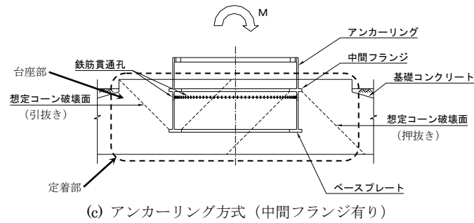
図-解 4.9.3 重力式構造におけるアンカー接合部の例 4)
