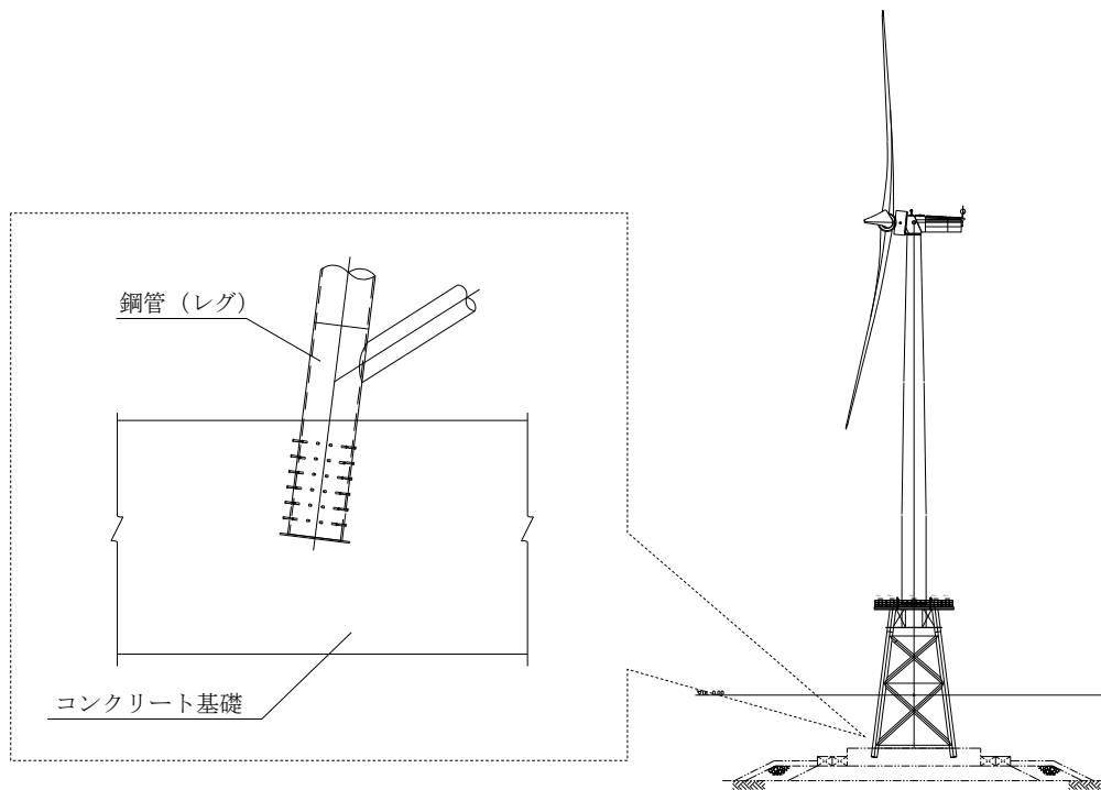
図-解 4.9.4 ジャケット構造とフーチング間の埋め込み接合の例
