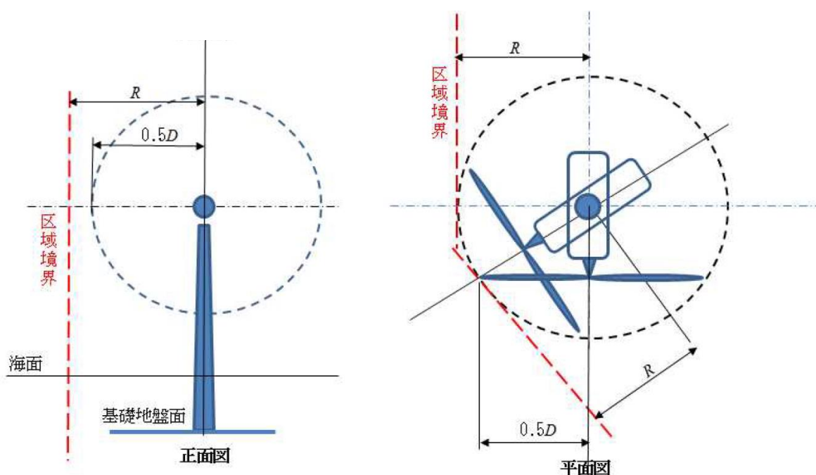
図-解 2.12.1 「再生可能エネルギー源を活用する区域」の境界と洋上風力発電設備の位置関係 1)
