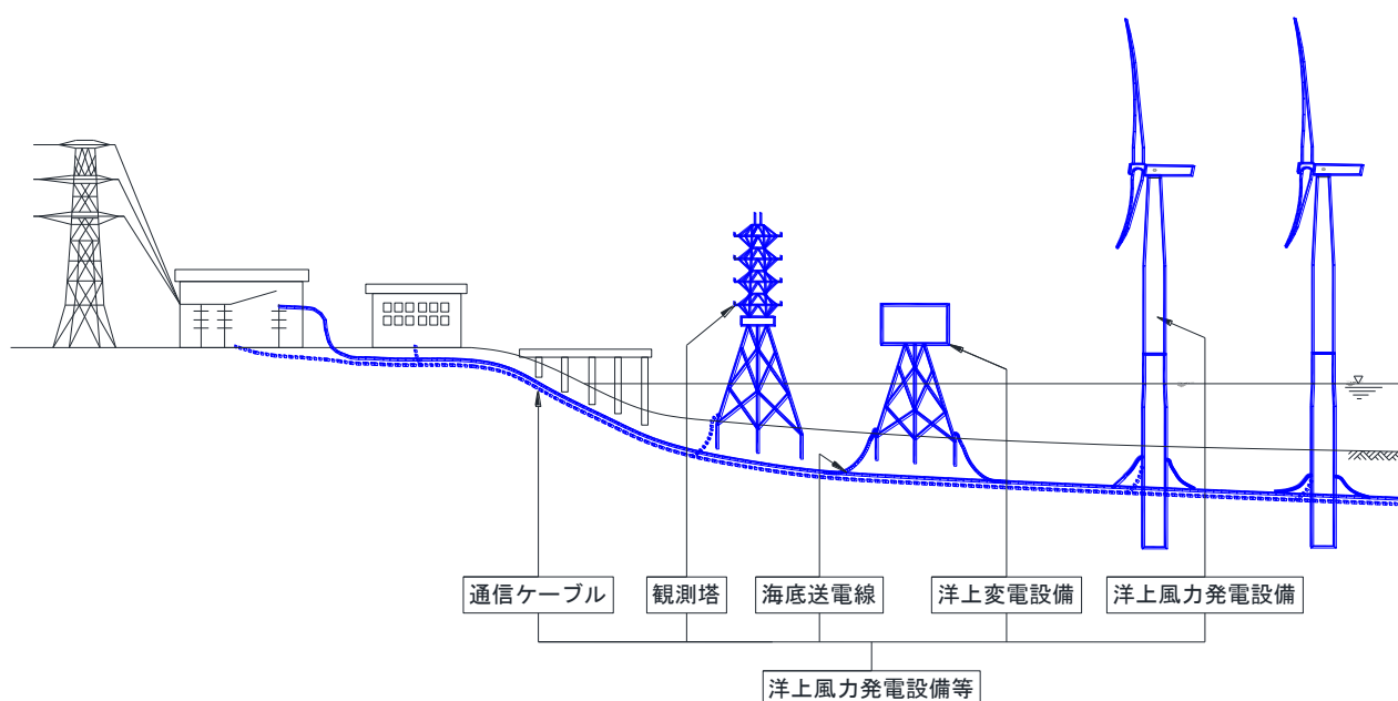
図-解 1.1.2 本基準解説の対象となる設備
