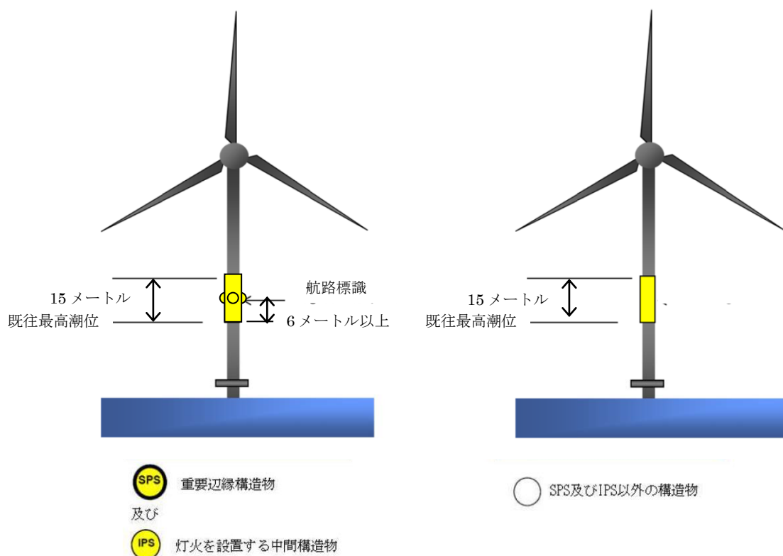
図-解 2.11.1 洋上風力発電設備等の塗色及び灯火の例 1)
