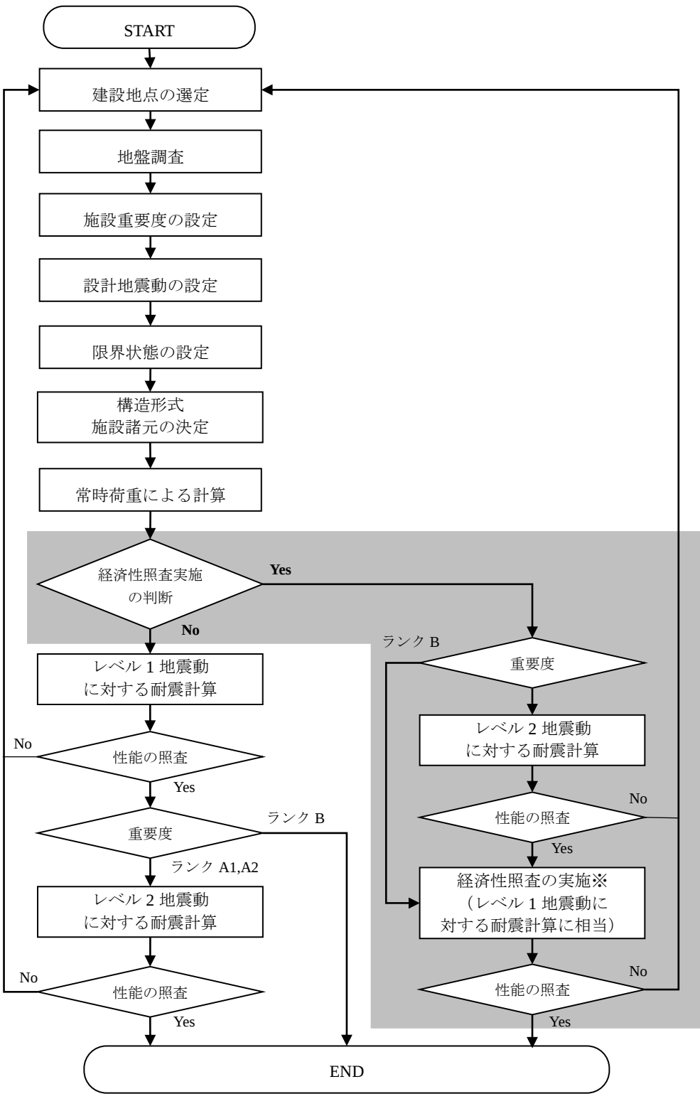
水道耐震工法指針（2022 年版）本編 図-3.1.2、p.26 に加筆 図 2.2 耐震設計のフロー（新設）
