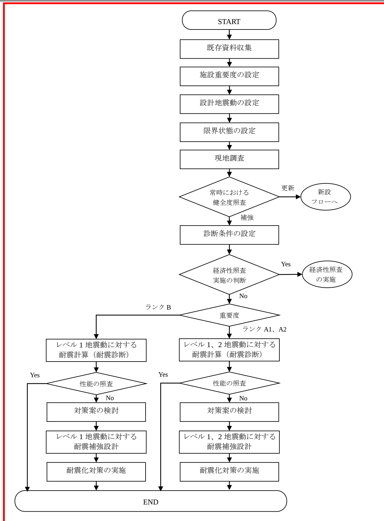
図 2.3 耐震設計のフロー（既設）
