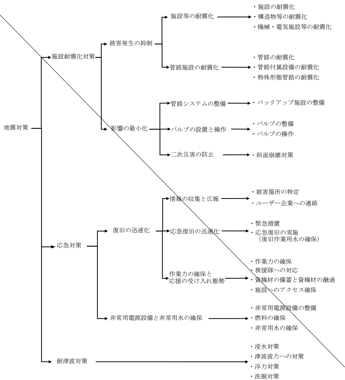
図 3.1 工業用水道における地震対策 (厚生労働省：水道の耐震化計画等策定指針の図-5 に加筆)
