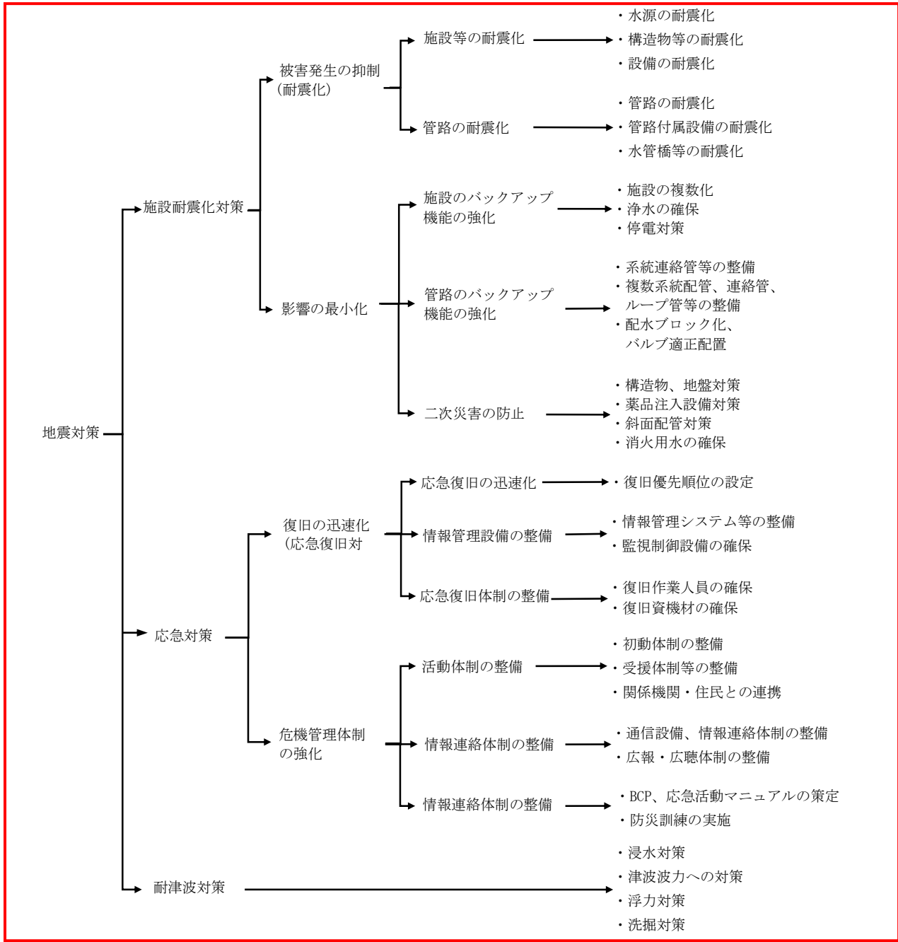
図 3.1 工業用水道における地震対策 (国土交通省：水道の耐震化計画等策定指針の図-5 に加筆)
