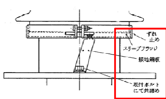
【遮断器】
