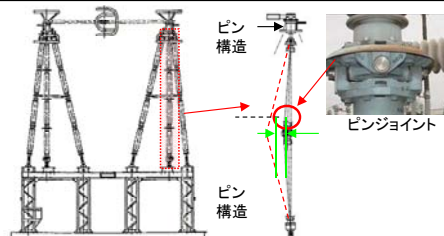
【遮断器】
