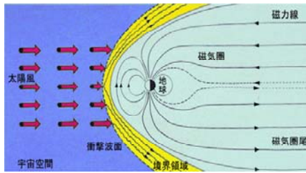
太陽フレアにより放出された高エネルギー粒子が磁気嵐の発端(例)
