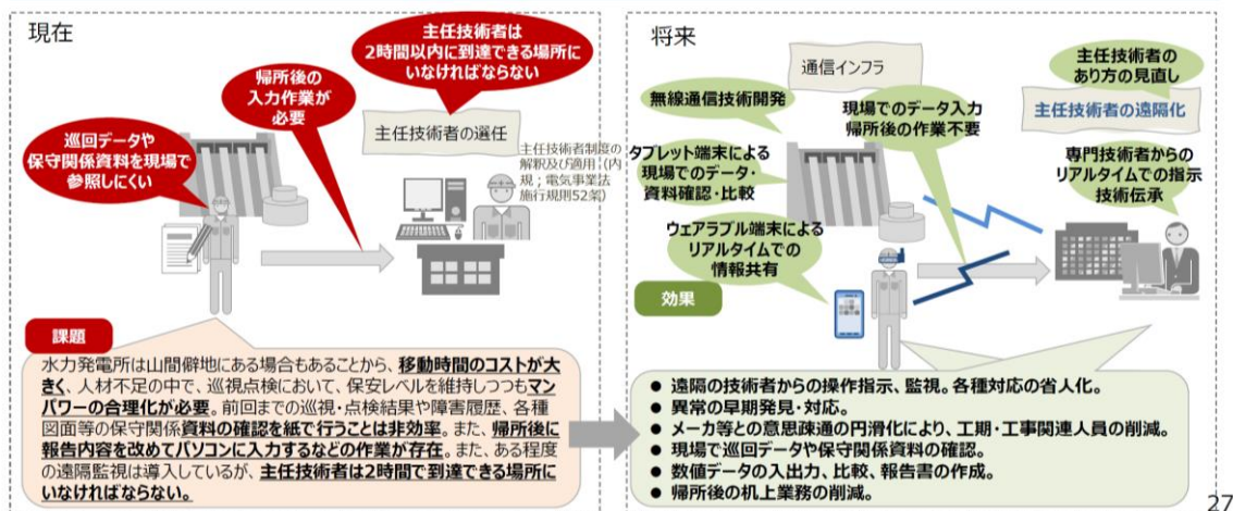
図 10 水力発電分野における技術（デジタル端末の活用による現場作業高度化）
