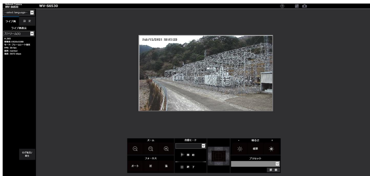
図 20 ネットワークカメラ本体（上図）および監視画面（下図）の例
