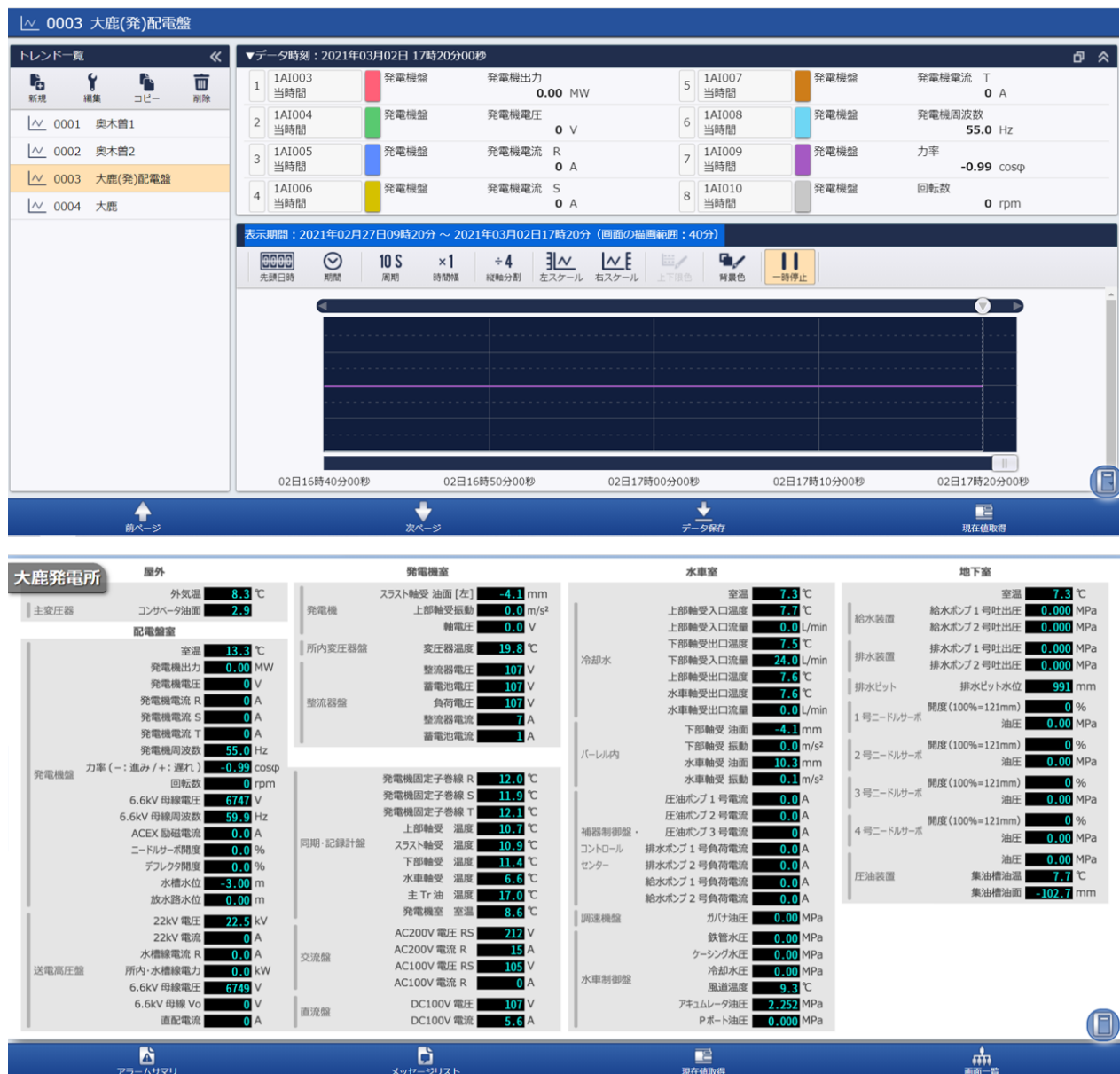
図 14 大鹿発電所の監視画面例
