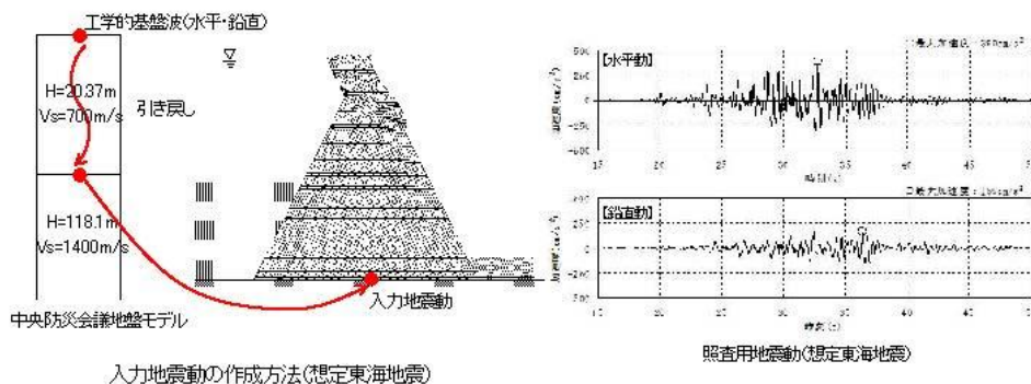
入力地震動の作成方法(想定東海地震)
