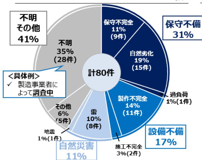
令和3～5年度の電気工作物の破損の原因内訳
