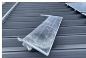
屋根上に飛散したモジュール 民家の庭に散乱したモジュール
