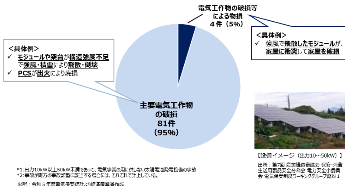
太陽電池発電設備（出力10kW以上50kW未満）の事故内訳【令和5年度】※1・2
