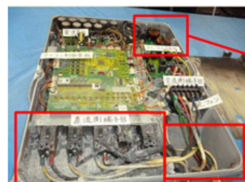
PCSの焼損事故の例
