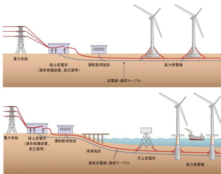
ウインドファームの主要構成要素（上：陸上 下：洋上）
