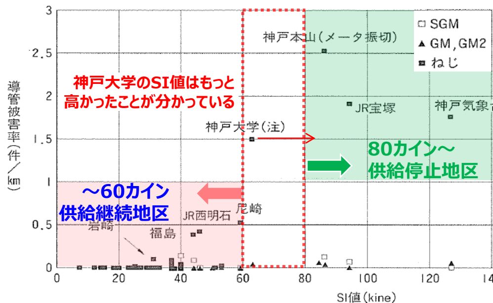
図 阪神・淡路大震災の導管被害率 (「ガス地震対策検討会報告書（1996年）」に加筆)
