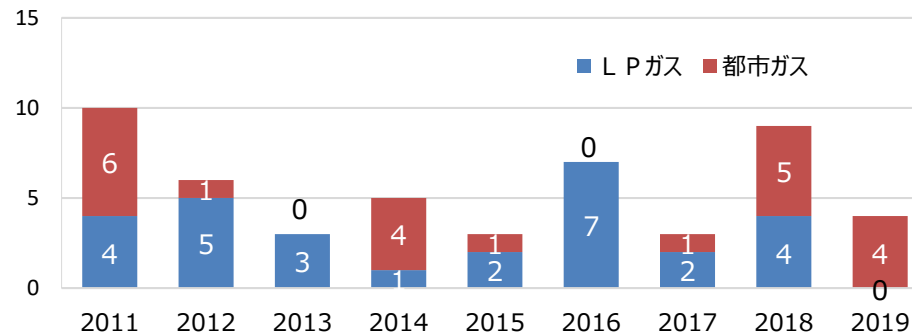
(件) 業務用厨房施設におけるCO中毒事故件数
