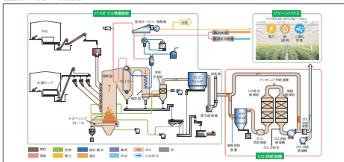
Fig.22 排ガス浄化・CO 2 供給設備フロー
