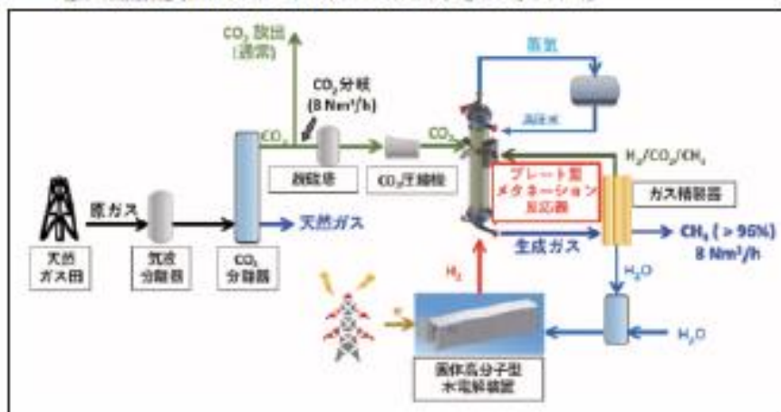
Fig.4 メタネーションによるカーボンリサイクル
