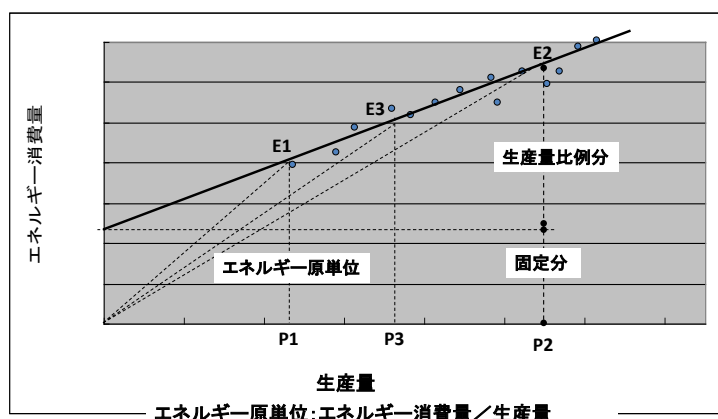
図 5. 生産量とエネルギー消費量との関係
