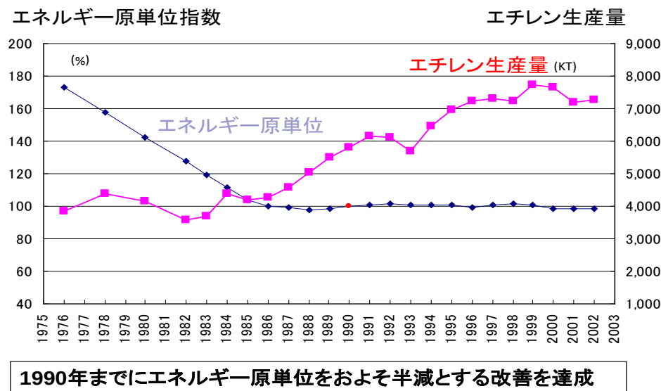
図 16. エチレン製造プロセスの原単位推移
