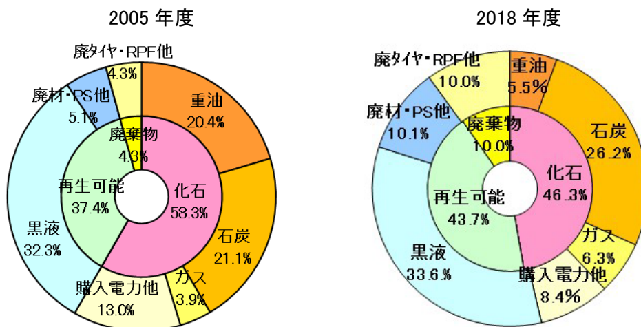
図3 エネルギー構成比率比較 (2005年度、2018年度比較)
