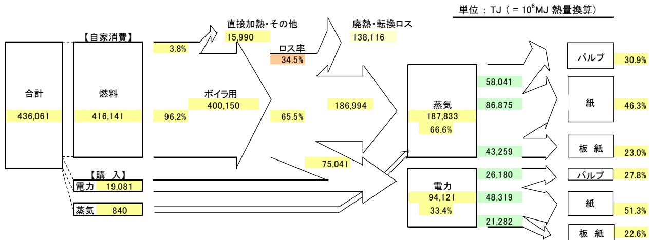
図8 紙パルプ産業のエネルギー消費バランス CY2018(平成30)年
