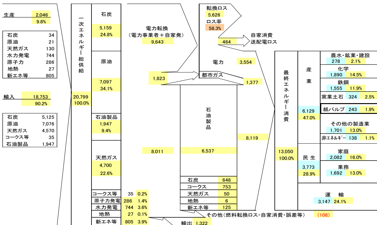
図7 我が国のエネルギーバランス CY2017(平成29)年
