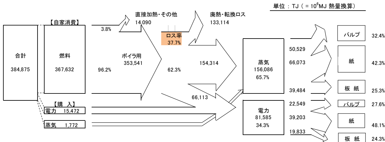
図10 紙パルプ産業のエネルギー消費バランス CY2020(令和2)年
