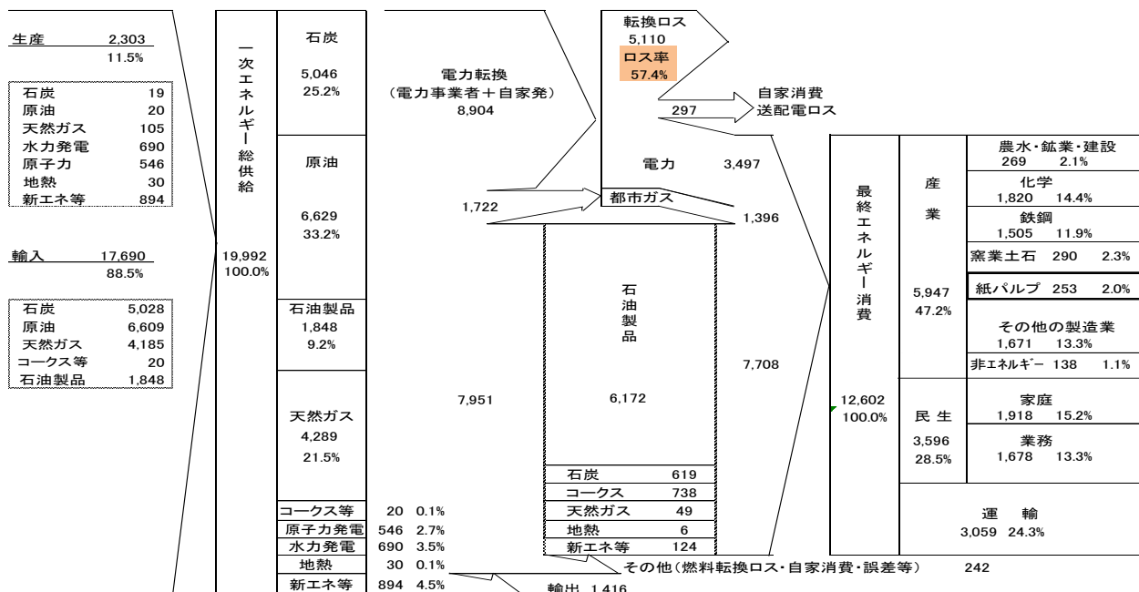
図9 我が国のエネルギーバランス CY2019(令和元年)
