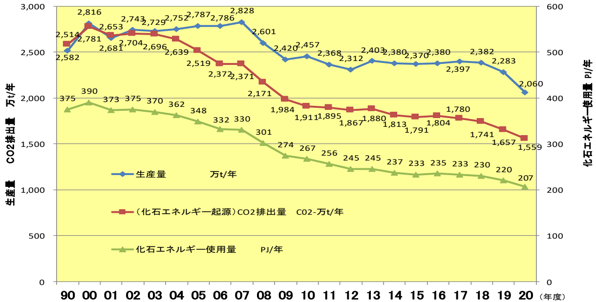
図1 生産量とCO 2 排出量および化石エネルギー使用量の推移
