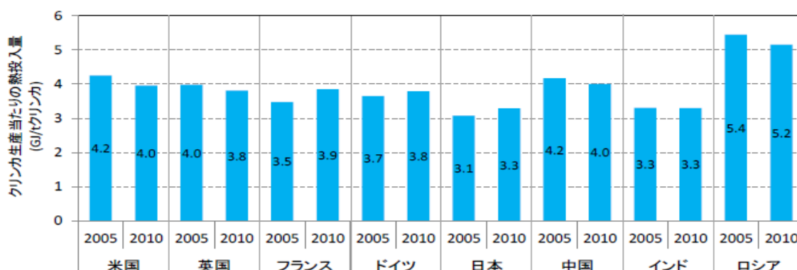
図 クリンカ製造の熱エネルギー原単位推計値(2005 年、2010 年)
