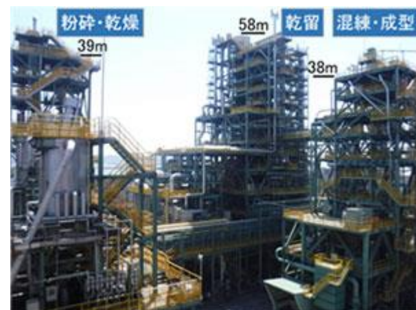
フェロコークス製造設備外観
