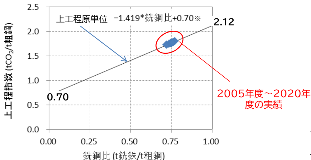
銑鋼比と上工程原単位の関係
