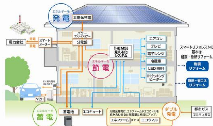
スマートリフォレスト イメージ図 (HEMS のメーカー・種類により、表示できる機器が異なります。)
