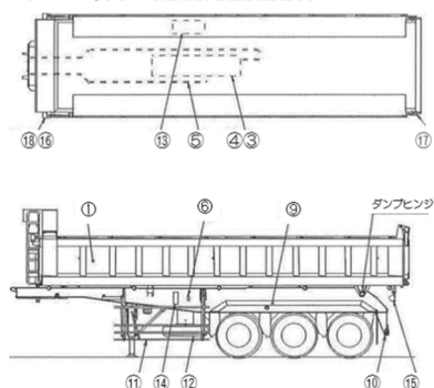
解体部品
