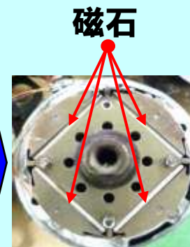
ロータ磁石
