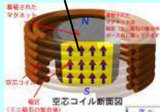
磁区の向き
