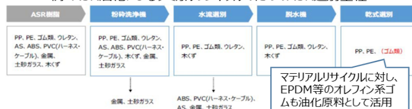
例 ASR油化によるケミカルリサイクルのためのASR選別工程
