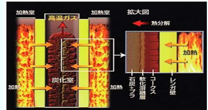
● コークス炉の構造と熱分解進行状況
