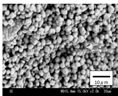
図 3-17. ランプ用スクラップのSEM観察
