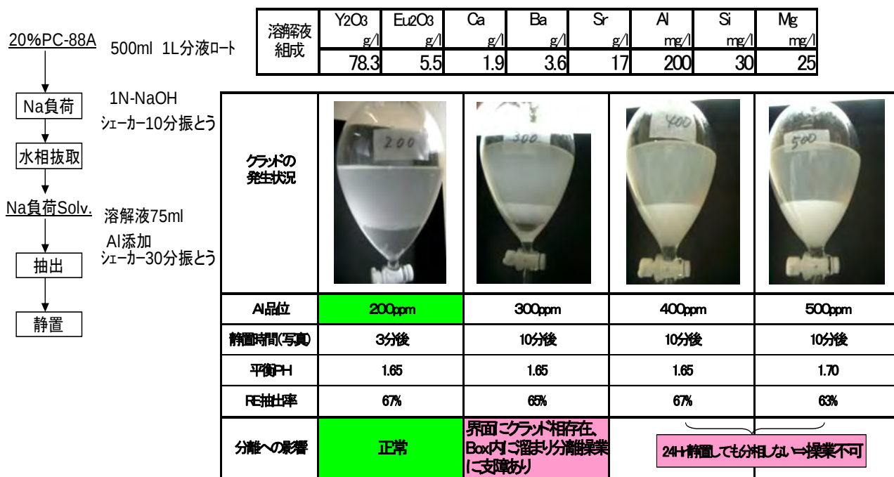
図 3-33. 不純物（A I）の抽出試験結果
