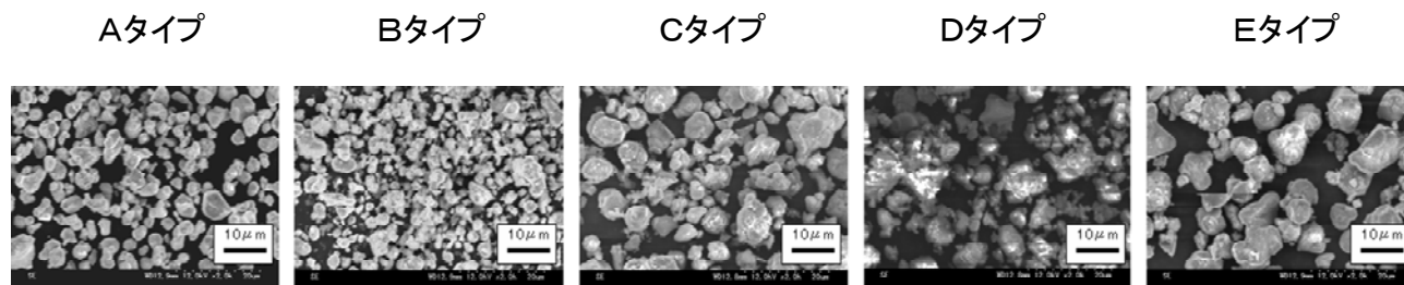
図 3-30. SEM観察結果
