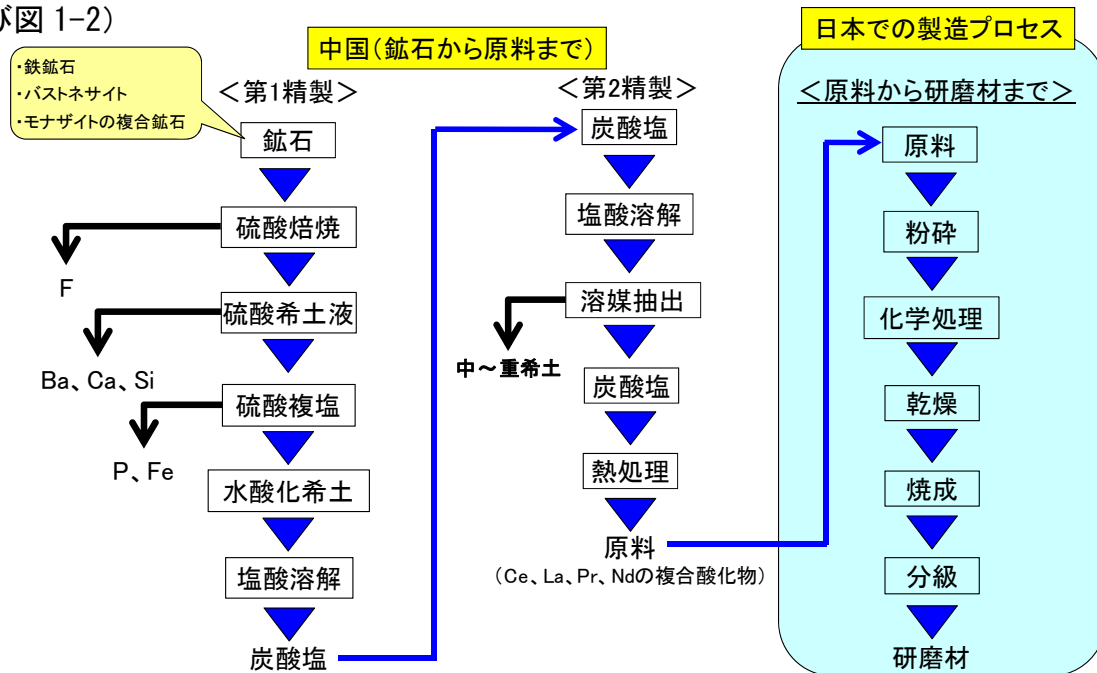
図1-1 原料から研磨材製品までの流れ
