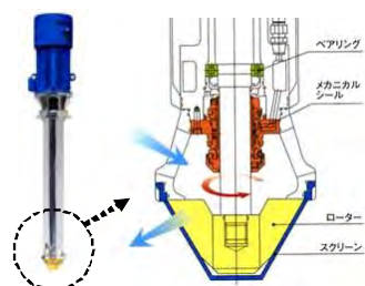
図3-11. 分散処理試験結果及びホモジナイザー概要図
