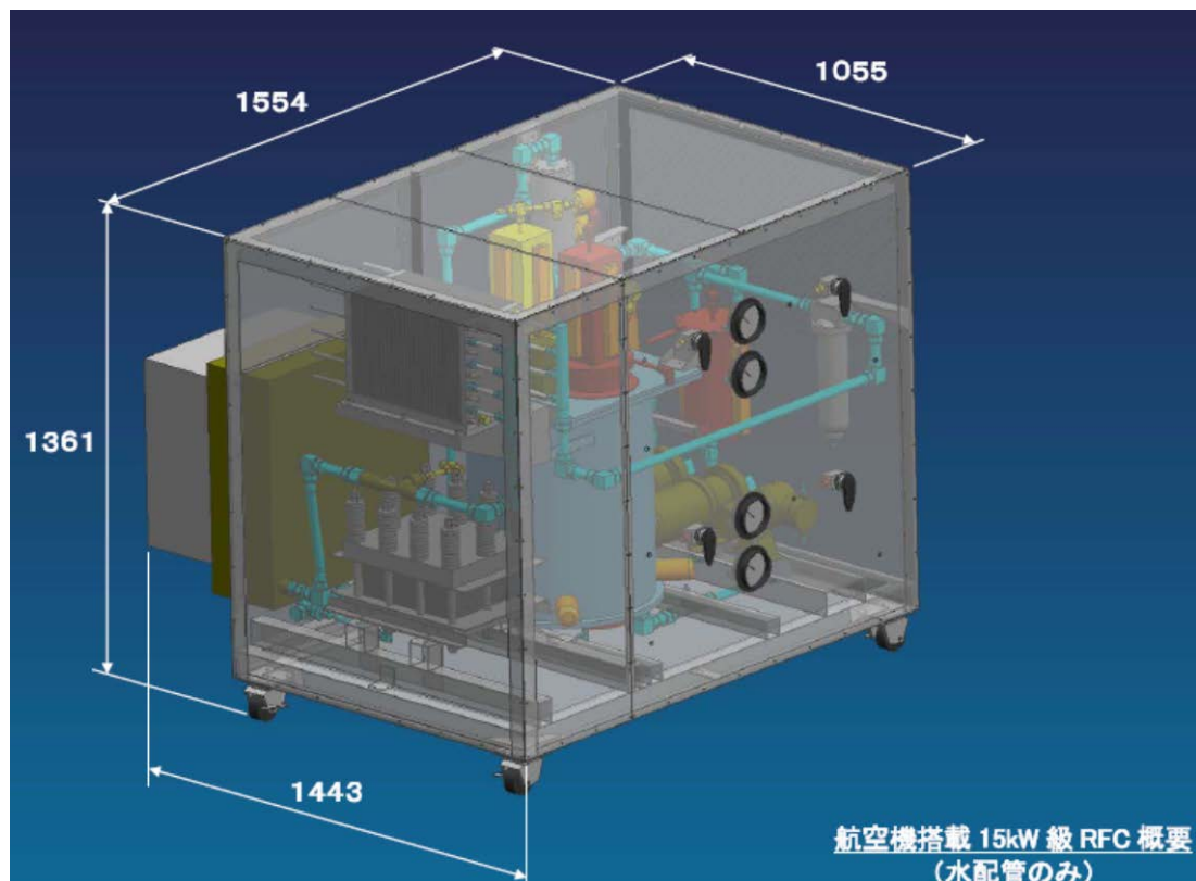
図 3. 15kW 級 RFC 原理確認モデル概観図
