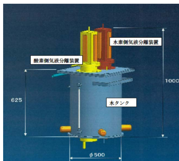
図2. 気液分離器概観図
