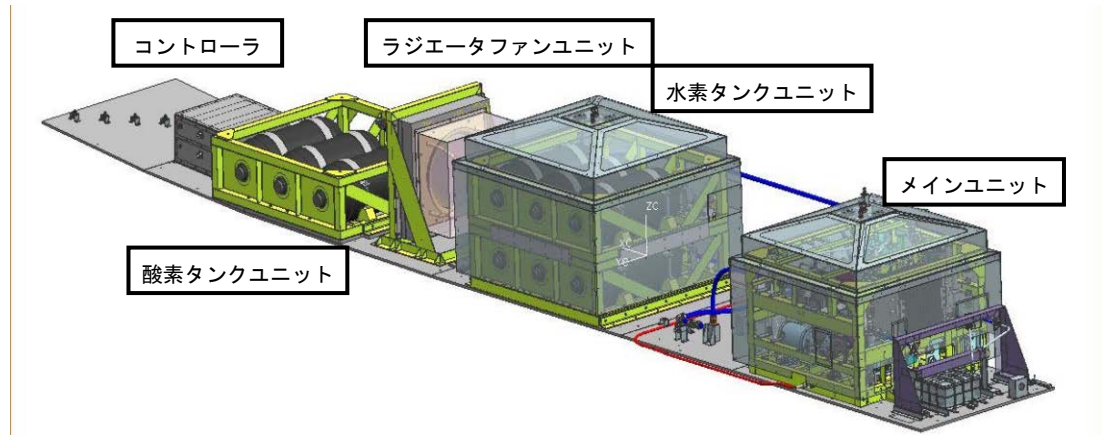
図5. RFCシステム概観図
