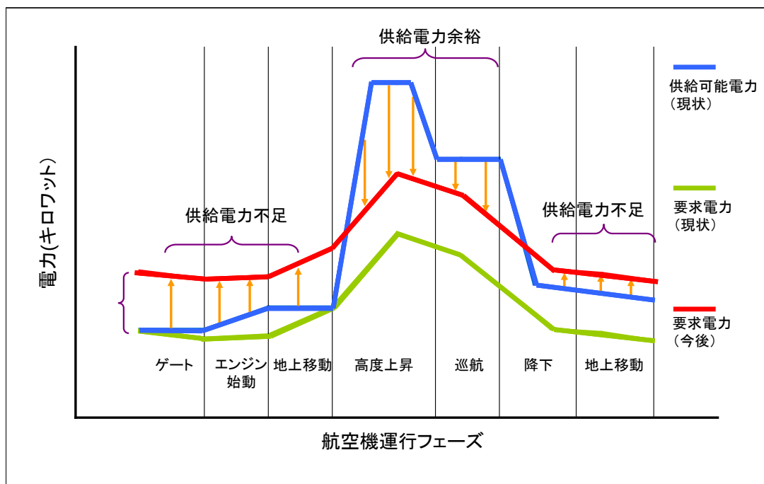
図1. 航空機での電力需要／供給プロファイル例
