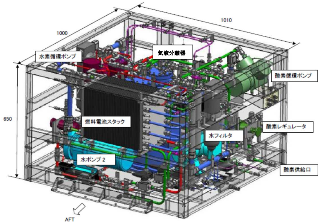
図４．ＲＦＣ小型化検討結果（メインユニット部）
