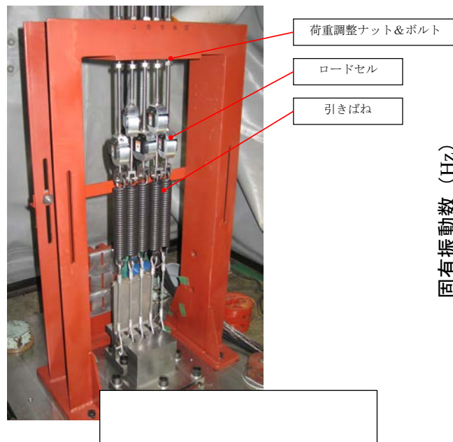
[1]-1 単翼ダンパ要素試験装置
