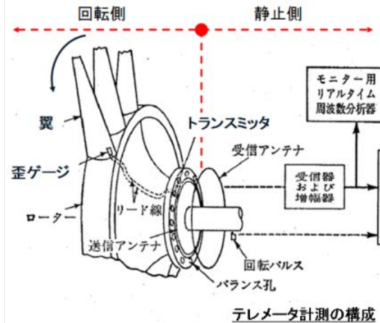
テレメータ計測の構成
