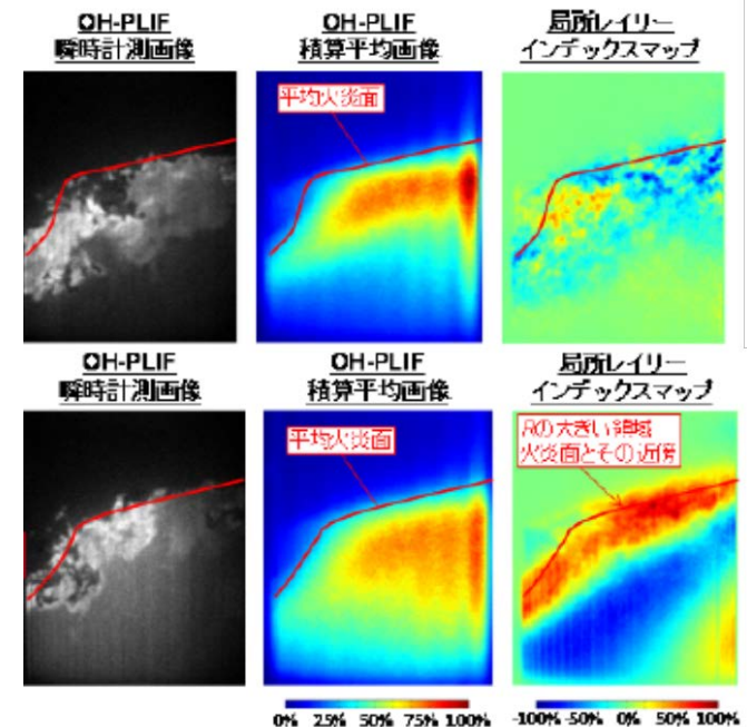
不安定燃焼領域の可視化
