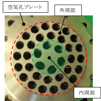
図 空気孔プレート
