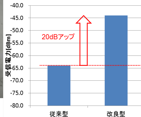
アンテナ改良による受信電力特性向上
