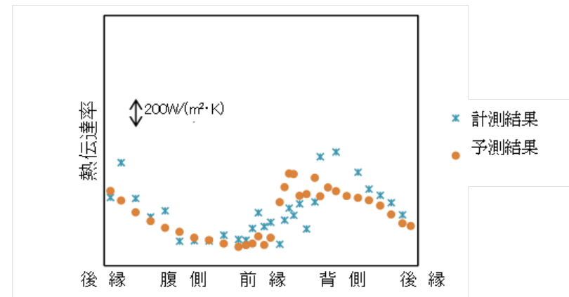
翼面熱伝達率分布
