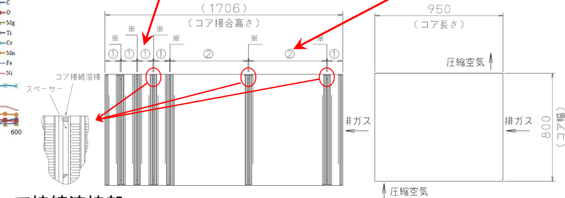
コア接続溶接部 断面(※)
