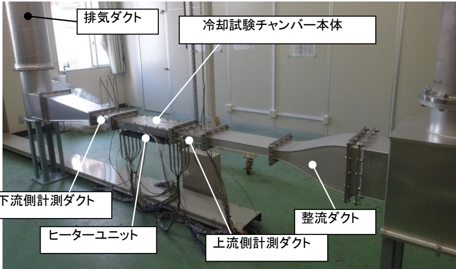
図 ライナ冷却要素試験装置
