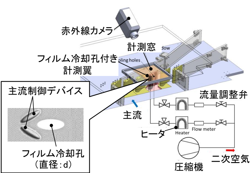
翼列風洞試験装置計測部
