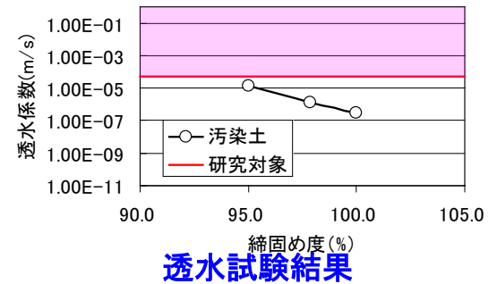
図 3-1-2(2)-5 鉛汚染土壌の物性
