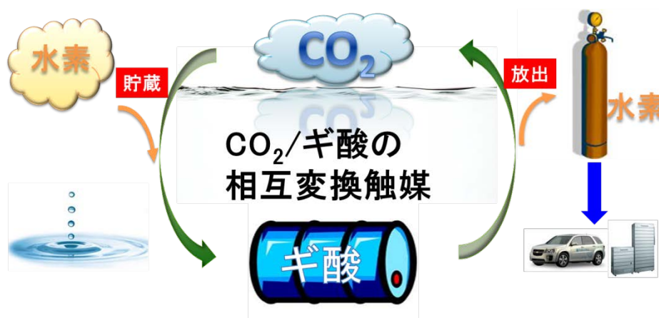
二酸化炭素とギ酸の相互変換による水素貯蔵技術のイメージ
